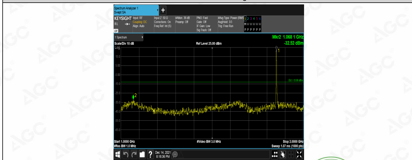
Band2-3MHz-QPSK-18615-1RB#0-Range2:1000~2000MHz
