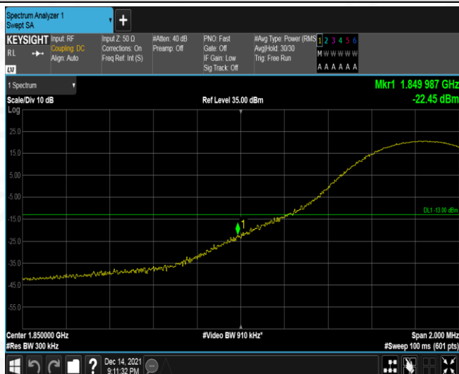
Band2-15MHz-QPSK-18675-1RB#74
