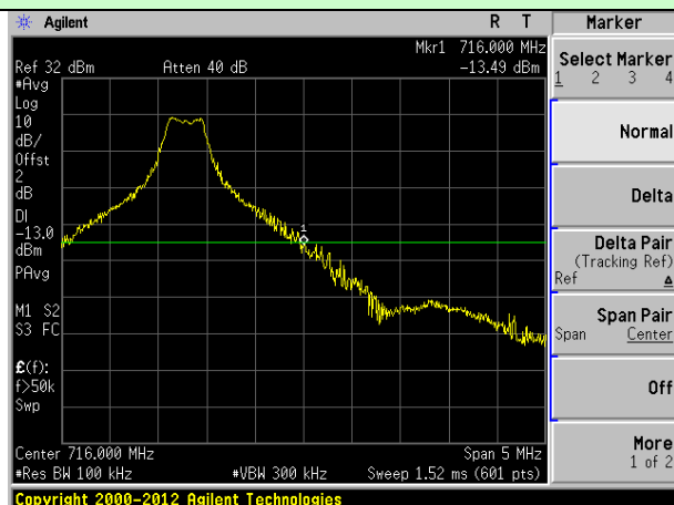
10MHz Bandwidth (RB size:1# RB offset:49#)
