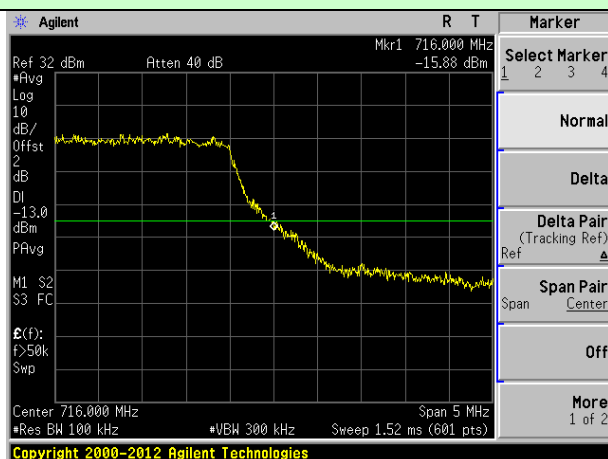
10MHz Bandwidth (RB size:25# RB offset:25#)
