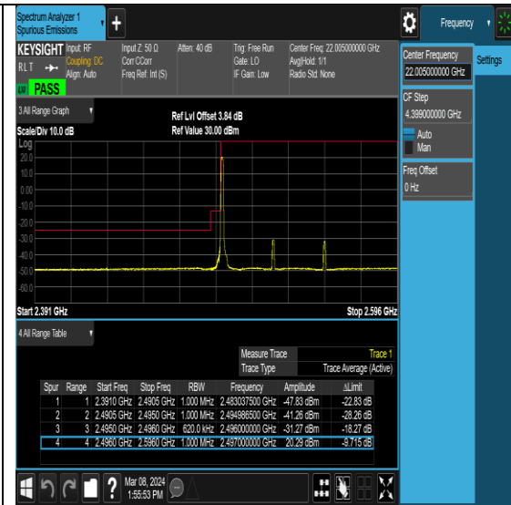
NTNV-N41-PC2-30-60-L-DFT-QPSK-Edge_1RB_Left-Ant0-PASS
