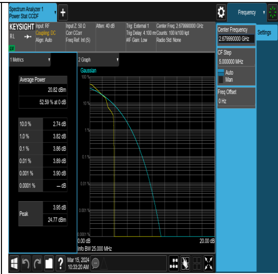
NTNV-N41-PC2-30-20-H-DFT-QPSK-Edge_1RB_Left-PASS
