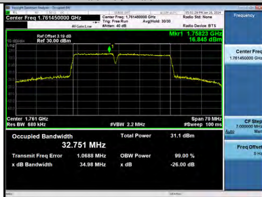
66-66-15MHz-20MHz-QPSK-QPSK-132401-132572-75R B#0-100RB#0-PASS
