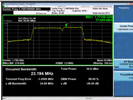
66-66-15MHz-10MHz-QPSK-QPSK-132499-132619-75R B#0-50RB#0-PASS
