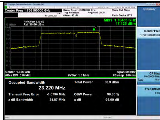
66-66-15MHz-10MHz-QPSK-QPSK-132373-132493-75R B#0-50RB#0-PASS
