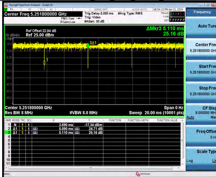
11AX20MIMO_Ant8_5260_52Tone_RU37
