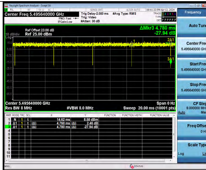
11AX20MIMO_Ant8_5500_26Tone_RU0
