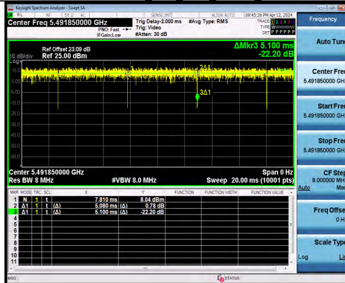
11AX20MIMO_Ant8_5500_52Tone_RU37
