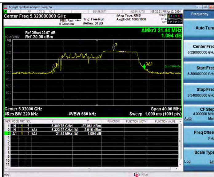
11AX20MIMO_Ant8_5320_26Tone_RU8
