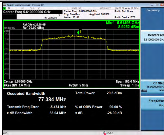
11AX80MIMO_Ant6_5690
