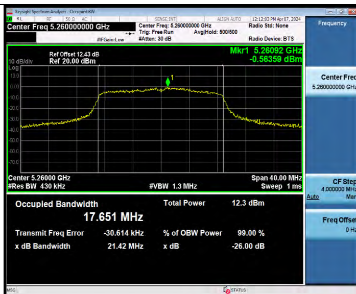
11N20MIMO_Ant8_5260
