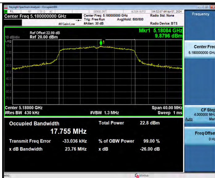
11N20MIMO_Ant8_5180
