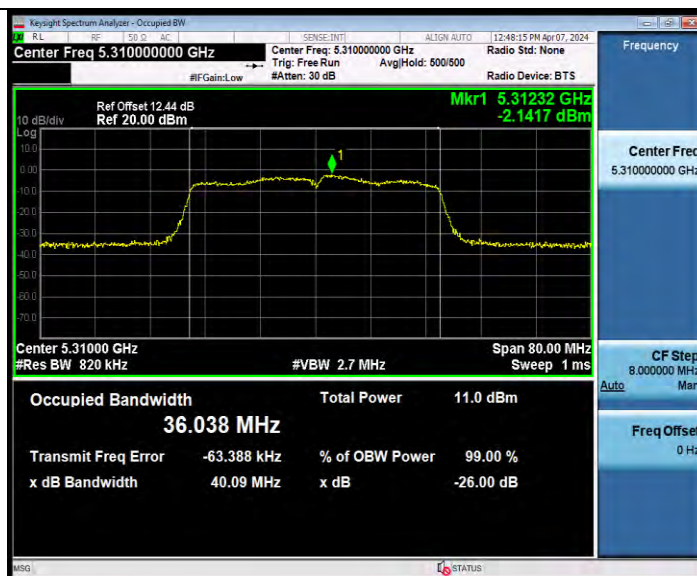
11N40MIMO_Ant8_5310
