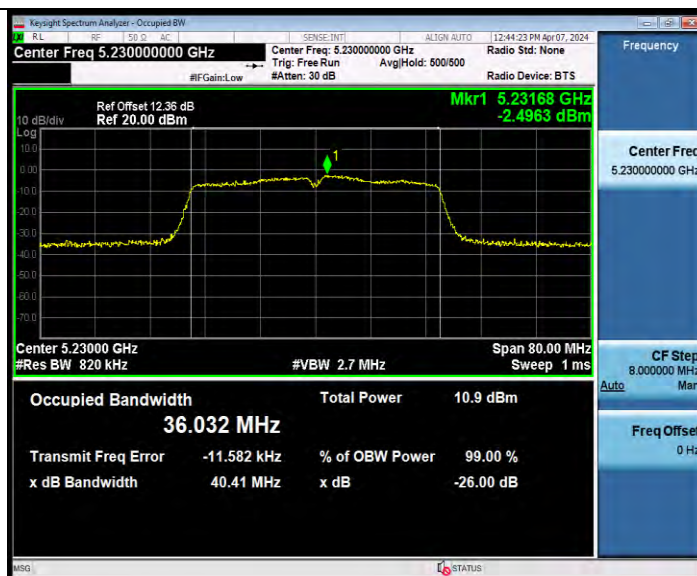
11N40MIMO Ant8 5230
