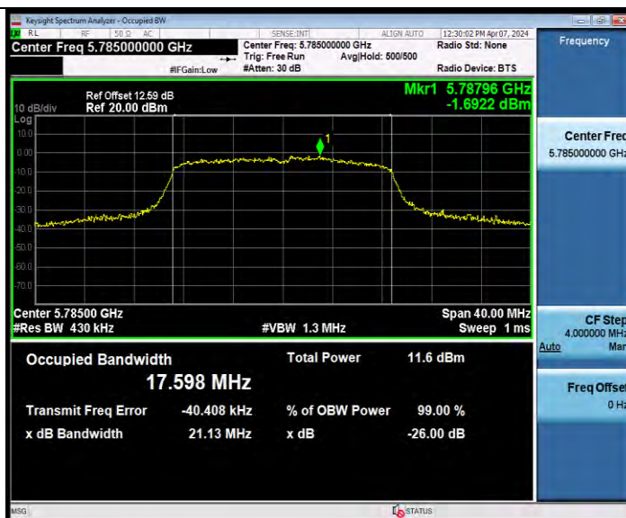
11N20MIMO_Ant8_5785
