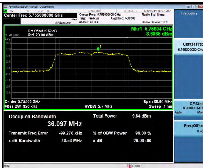
11N40MIMO_Ant8_5755
