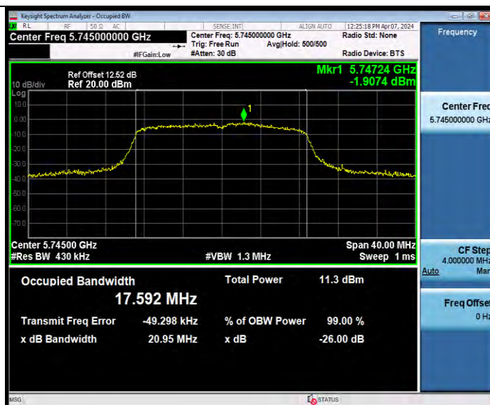
11N20MIMO_Ant8_5745
