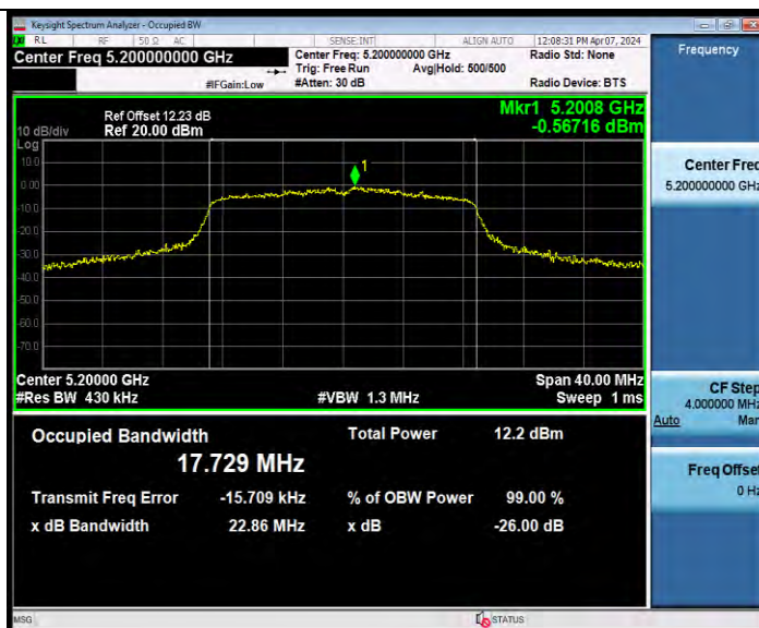
11N20MIMO_Ant8_5200
