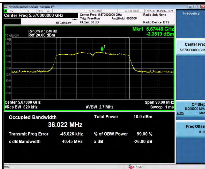
11N40MIMO_Ant8_5670
