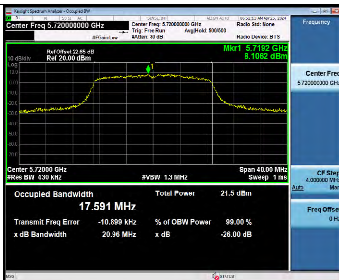
11N20MIMO_Ant8_5720
