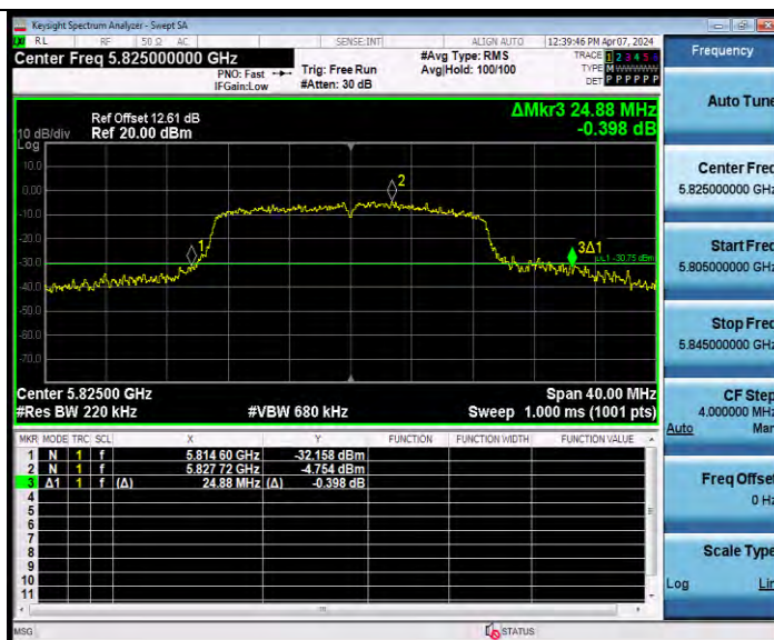
11N20MIMO Ant8 5825
