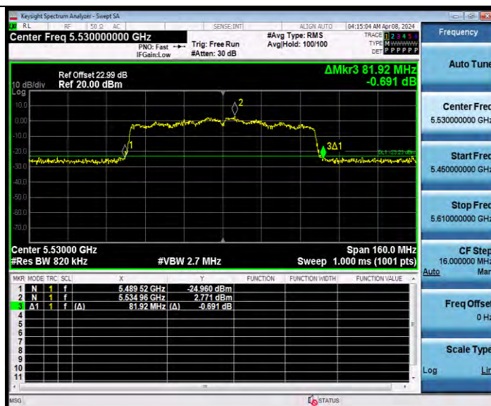
11AC80MIMO_Ant8_5530
