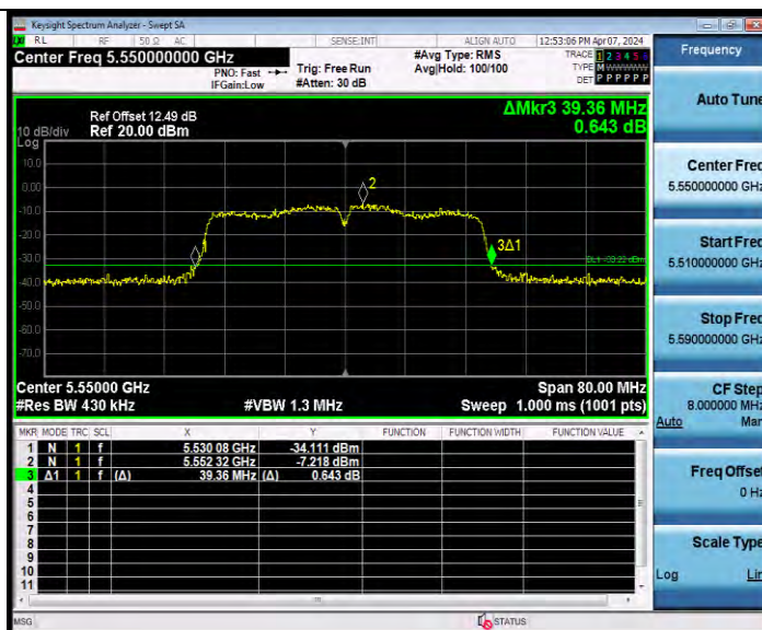
11N40MIMO Ant8 5550
