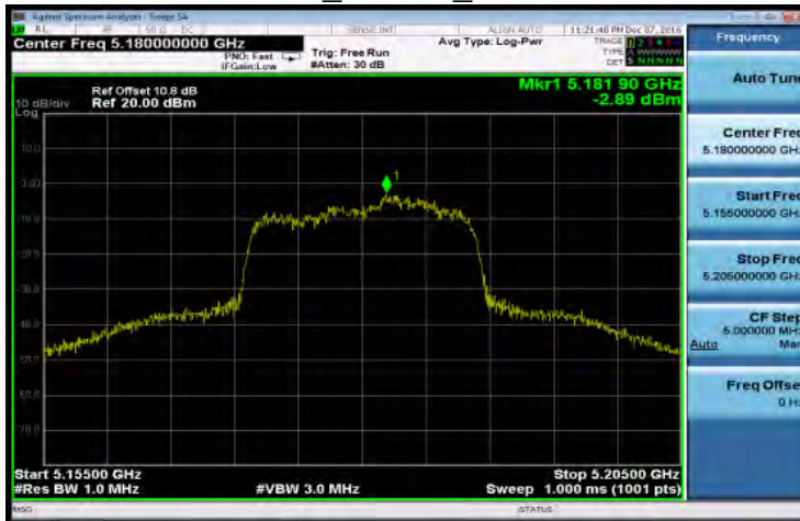
802.11a_20MHz_5180MHz
