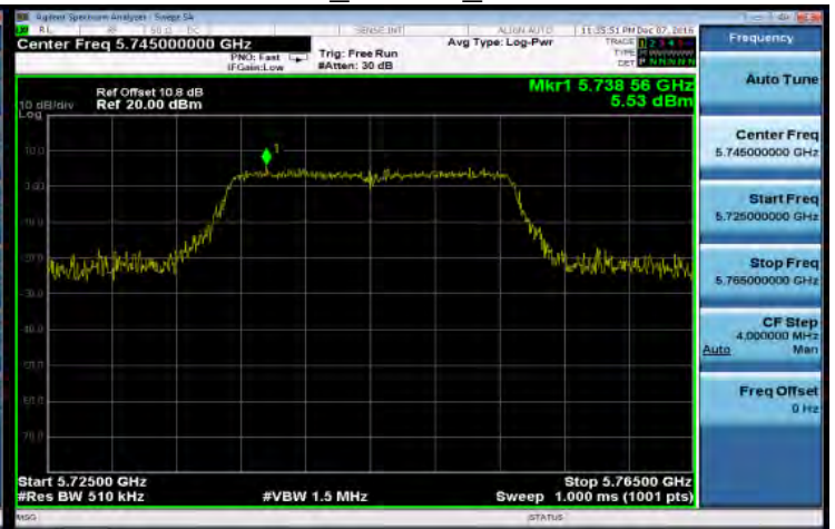
802.11n_20MHz_5745MHz
