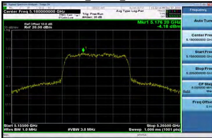
802.11n_20MHz_5180MHz
