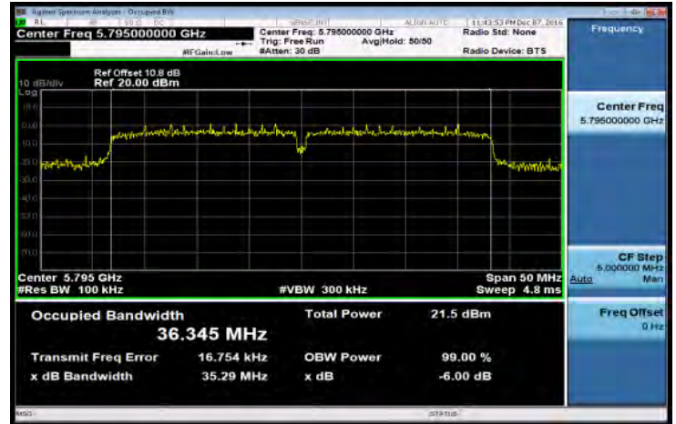
FCC_802.11n_40MHz_Main_5795MHz
