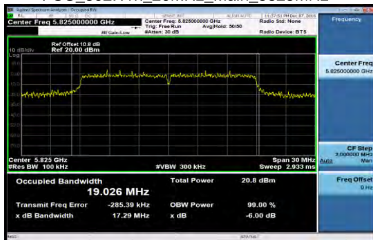
FCC_802.11n_20MHz_Main_5825MHz
