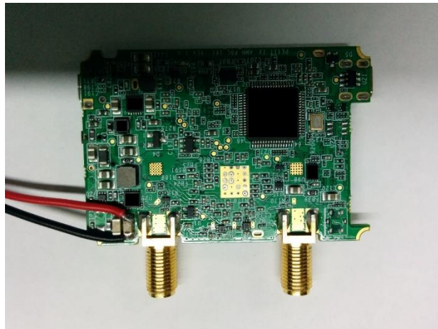
Figure 5 - VQSAMNPTTX01 (Variant: Petit) - Bottom View
