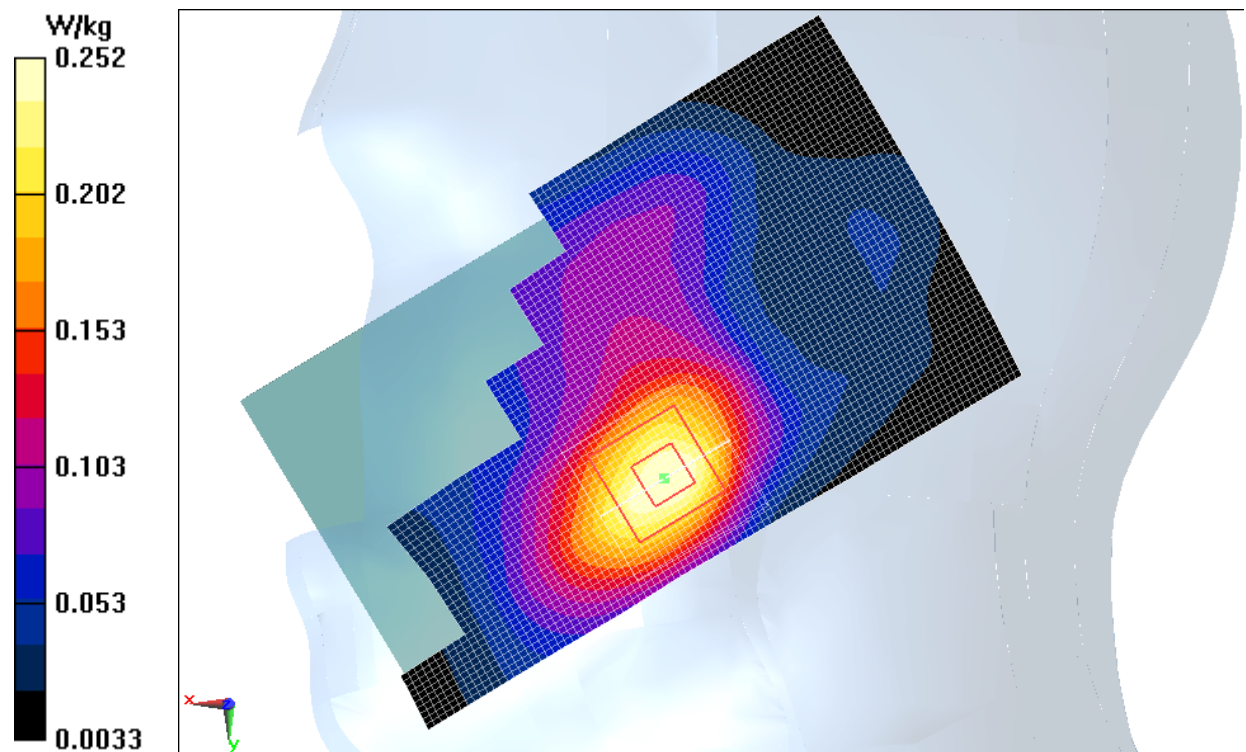
Fig.7 WCDMA1900 CH9538
