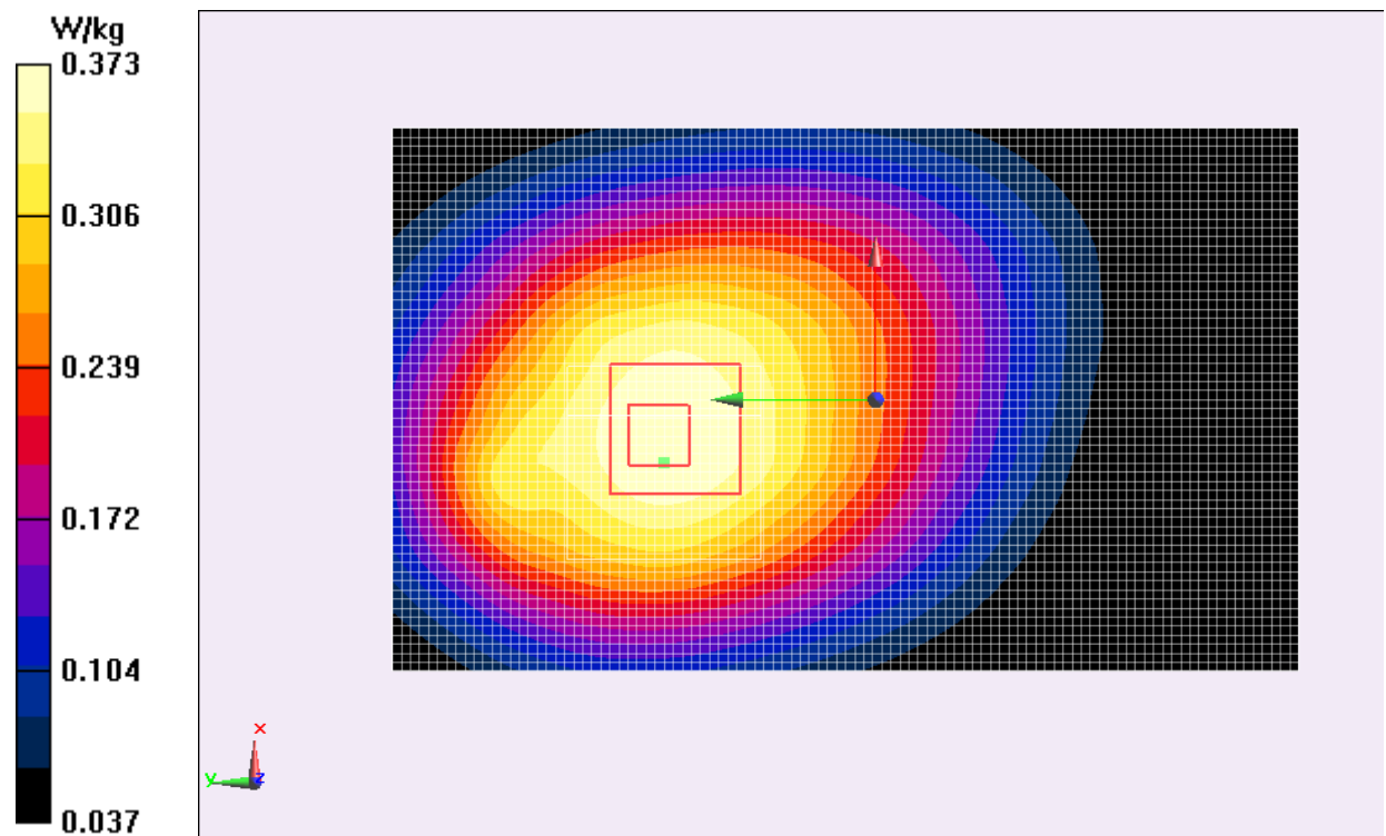
Fig.6 WCDMA 850
