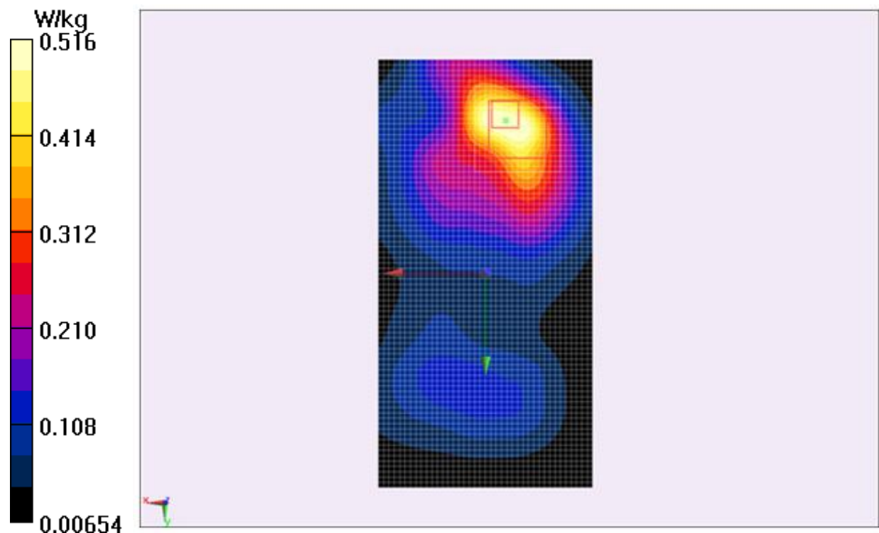
Fig.8 WCDMA1900 CH9262
