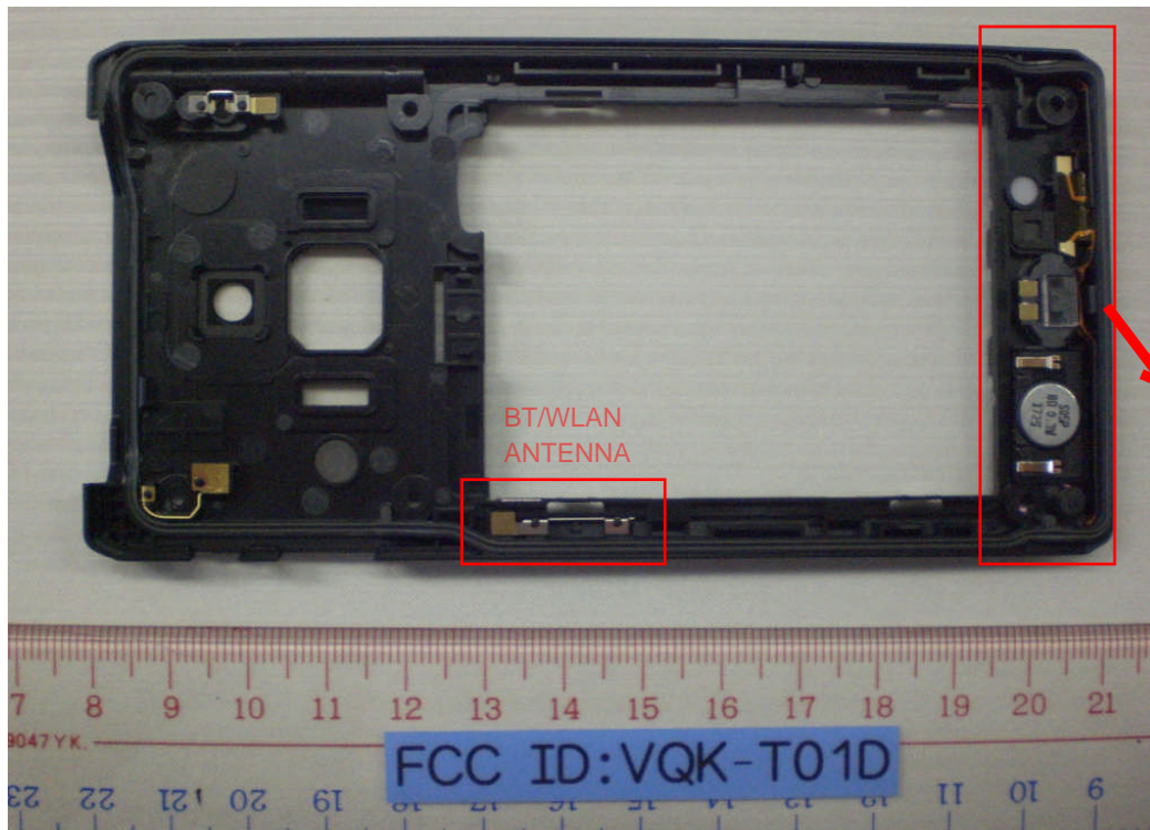
GSM/WCDMA ANTENNA
