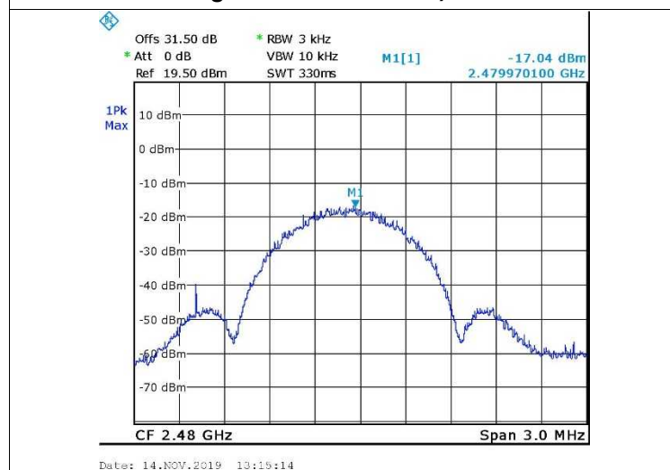
Figure 32. 2480.0 MHz, BLE
