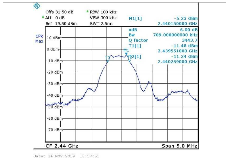
Figure 17. 2440.0 MHz, BLE
