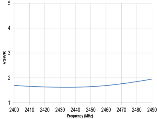
2.4 GHz VSWR
