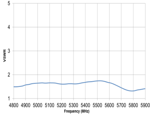
5 GHz VSWR
