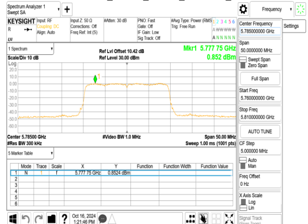
802.11ax_20MHz_Chain0_5785MHz_SU
