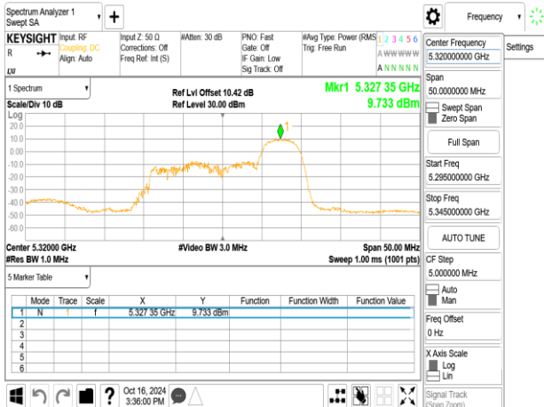
802.11ax_20MHz_Chain0_5320MHz_RU106_53
