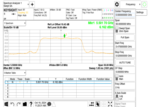
802.11ax_20MHz_Chain0_5500MHz_SU
