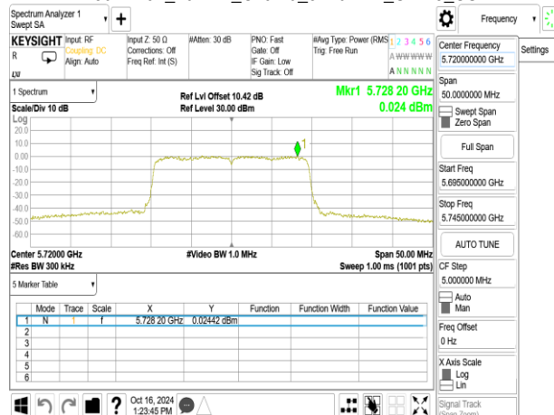
802.11ax_20MHz_Chain0_5720MHz_UNII 3_SU
