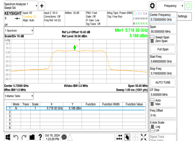
802.11ax_20MHz_Chain0_5720MHz_UNII 3_SU
