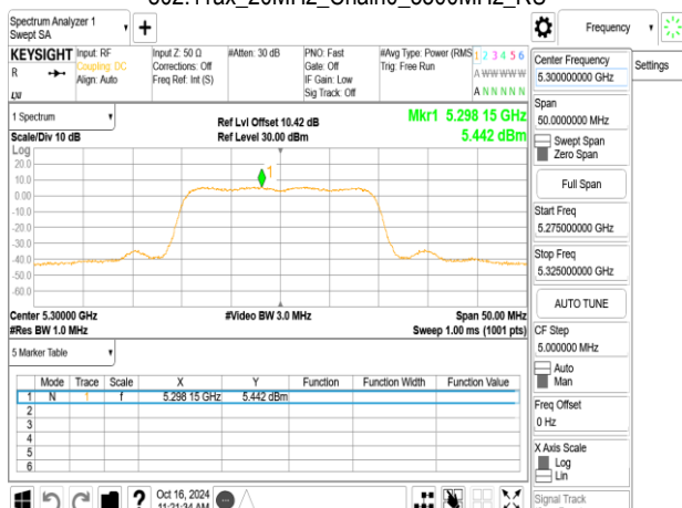
802.11ax_20MHz_Chain0_5300MHz_SU
