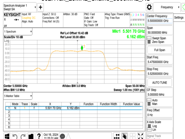
802.11ax_20MHz_Chain0_5500MHz_SU
