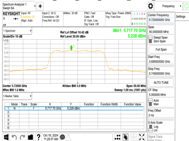
802.11ax_20MHz_Chain0_5720MHz_UNII 3_RU
