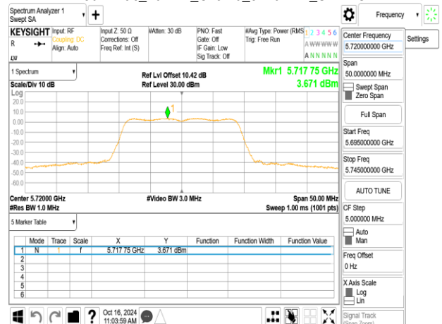
802.11ac_20MHz_Chain0_5720MHz_UNII 2C
