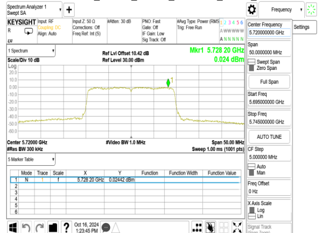
802.11ax_20MHz_Chain0_5720MHz_UNII 3_SU
