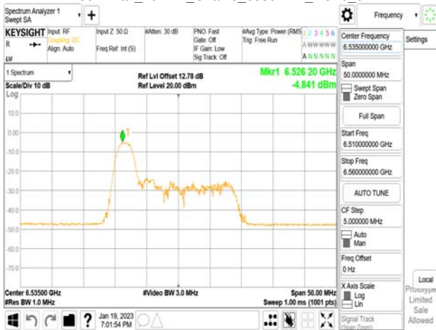
802.11ax_20MHz_Chain0_6535MHz_RU52_37
