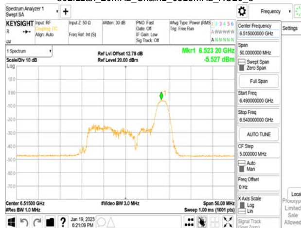
802.11ax_20MHz_Chain1_6515MHz_RU52_40
