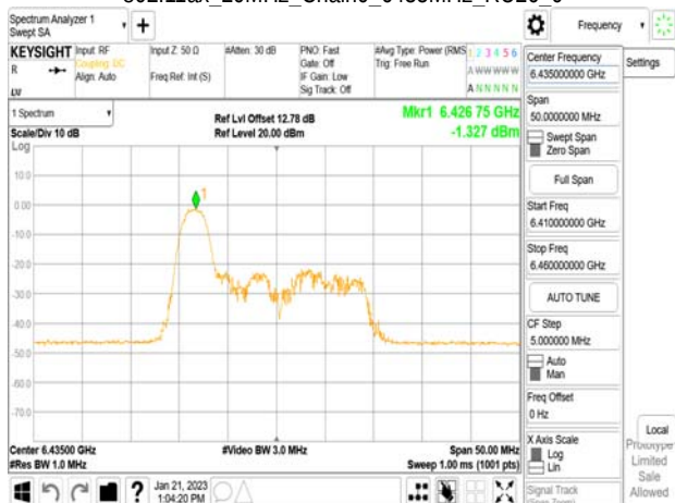
802.11ax_20MHz_Chain0_6435MHz_RU52_37
