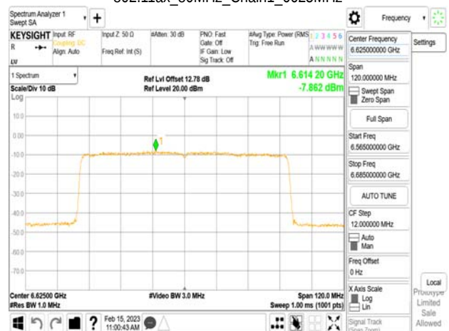
802.11ax_80MHz_Chain1_6625MHz
