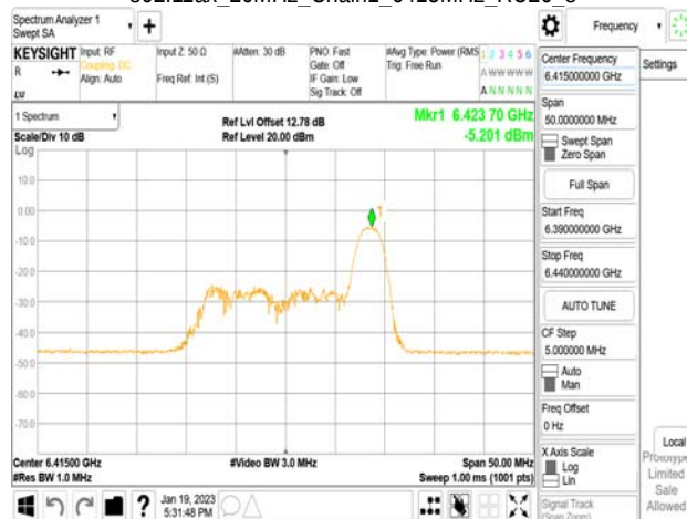
802.11ax_20MHz_Chain1_6415MHz_RU52_40
