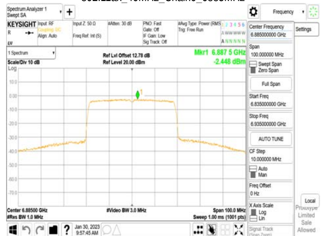
802.11ax_40MHz_Chain0_6885MHz
