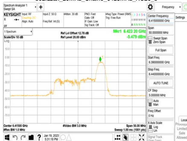
802.11ax_20MHz_Chain0_6415MHz_RU52_40
