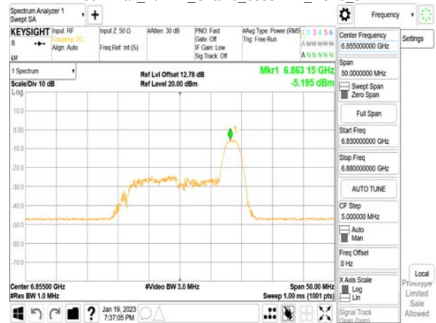
802.11ax_20MHz_Chain0_6855MHz_RU52_40
