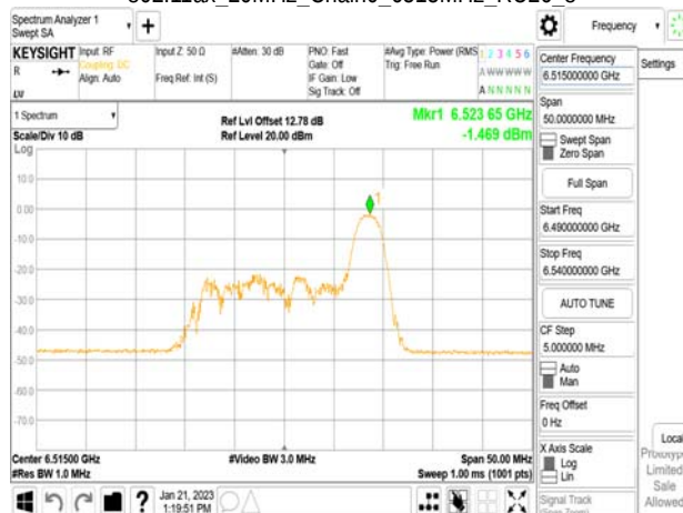
802.11ax_20MHz_Chain0_6515MHz_RU52_40
