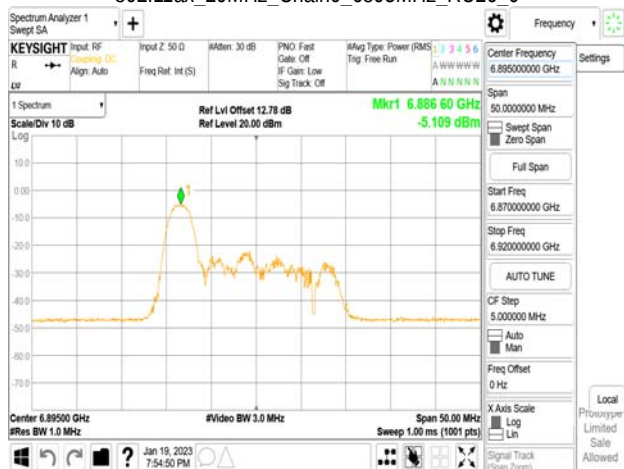
802.11ax_20MHz_Chain0_6895MHz_RU52_37
