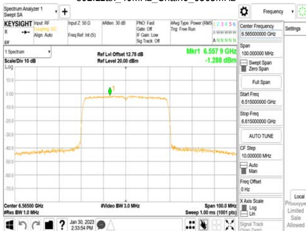
802.11ax_40MHz_Chain0_6565MHz
