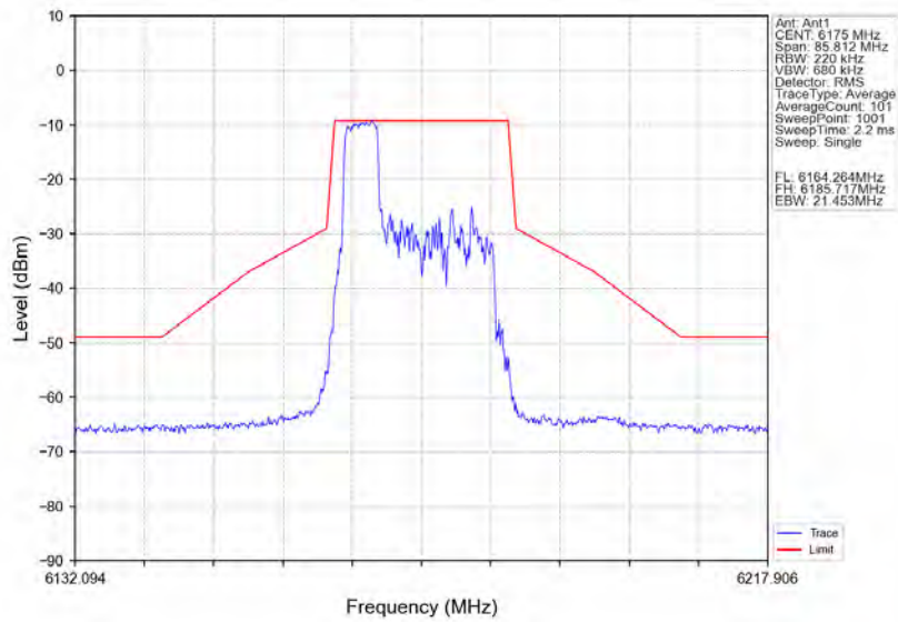
802.11ax(HE20)_MCH_6175MHz_RU52_Right_Ant1_NTNV
