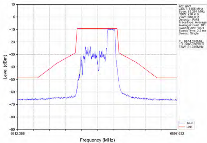
802.11ax(HE20) HCH_6855MHz_RU52_Right_Ant1_NTNV
