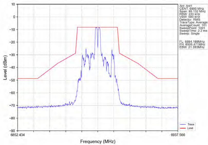
802.11ax(HE20)_LCH_6895MHz_RU26_Right_Ant1_NTNV
