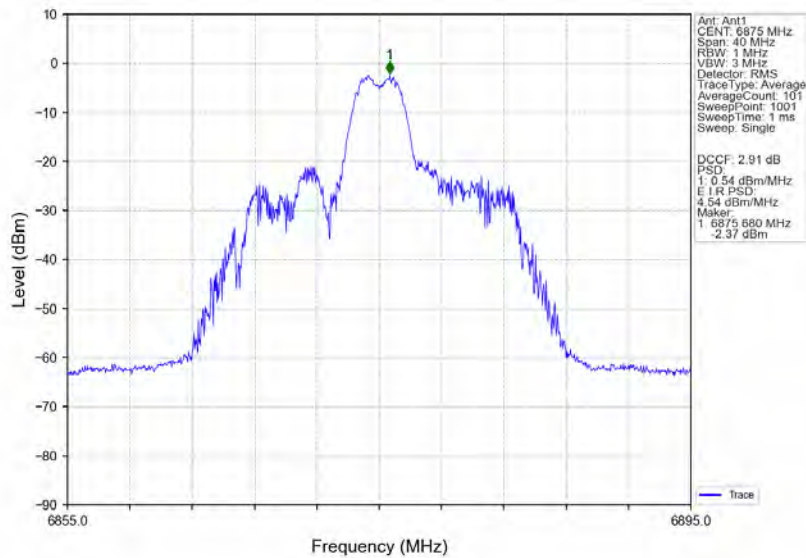
802.11ax(HE20) HCH_6875MHz_RU26_Right_Ant1_NTNV
