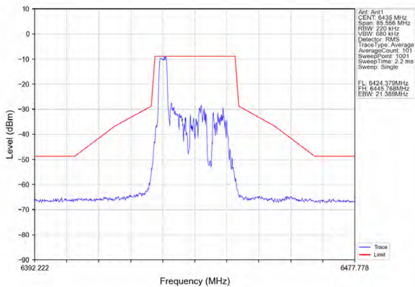
802.11ax(HE20)_LCH_6435MHz_RU26_Left_Ant1_NTNV
