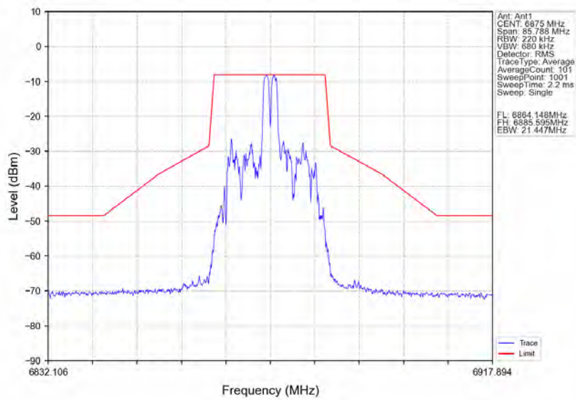
802.11ax(HE20) HCH_6875MHz_RU26_Right_Ant1_NTNV
