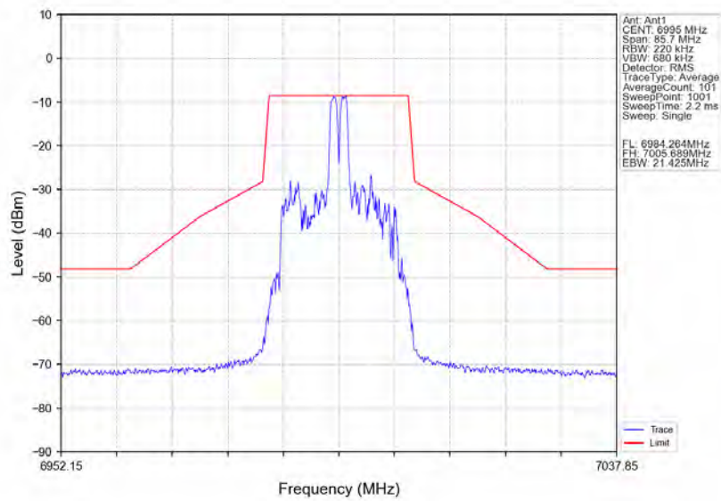
802.11ax(HE20)_MCH_6995MHz_RU26_Right_Ant1_NTNV
