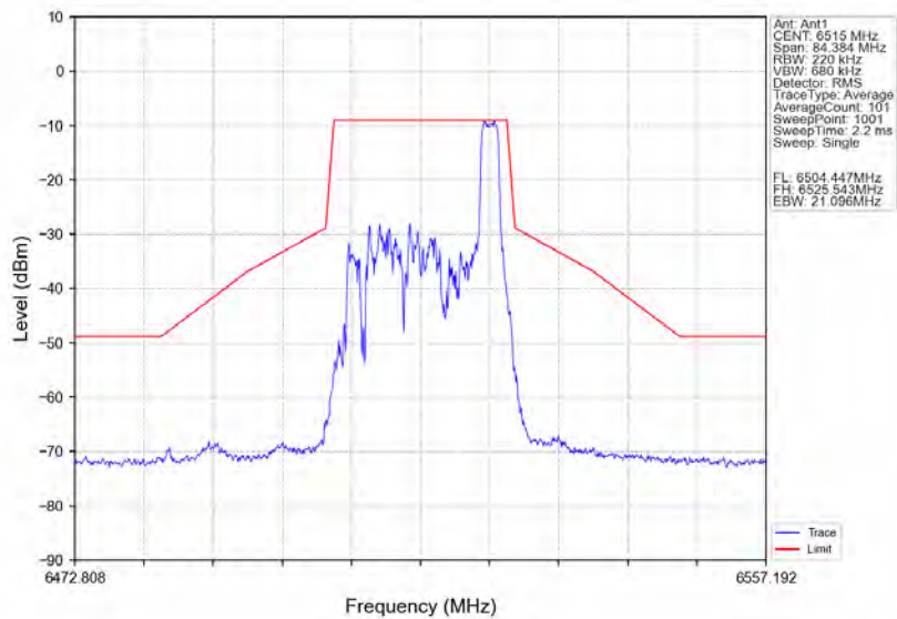
802.11ax(HE20) HCH_6515MHz_RU26_Right_Ant1_NTNV
