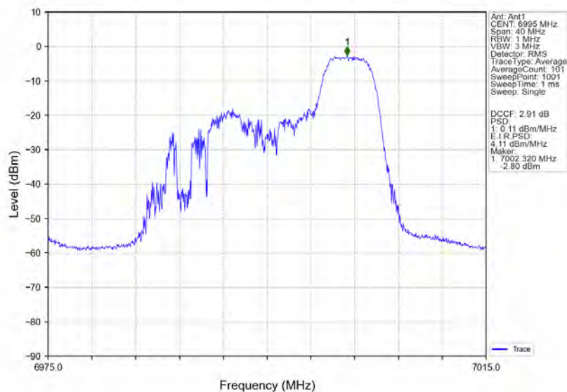
802.11ax(HE20)_MCH_6995MHz_RU52_Right_Ant1_NTNV
