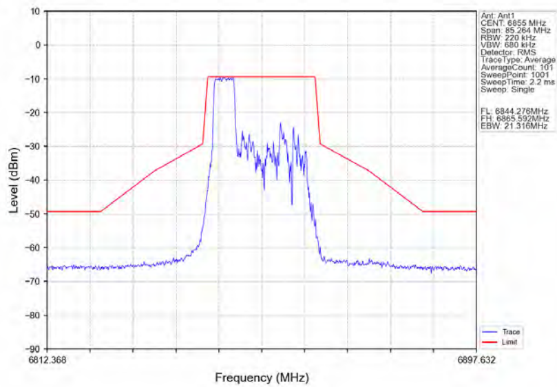
802.11ax(HE20) HCH_6855MHz_RU52_Right_Ant1_NTNV
