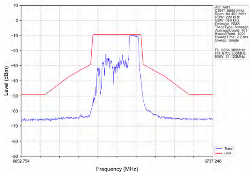
802.11ax(HE20)_MCH_6695MHz_RU52_Right_Ant1_NTNV
