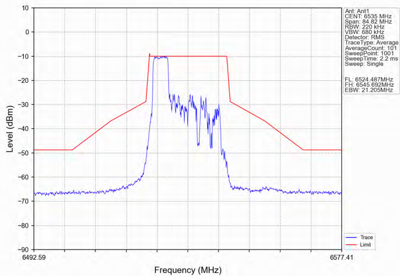
802.11ax(HE20)_LCH_6535MHz_RU52_Right_Ant1_NTNV
