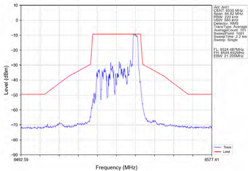
802.11ax(HE20)_LCH_6535MHz_RU26_Right_Ant1_NTNV
