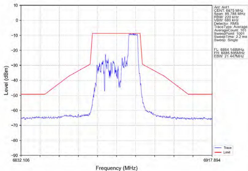
802.11ax(HE20) HCH_6875MHz_RU52_Right_Ant1_NTNV
