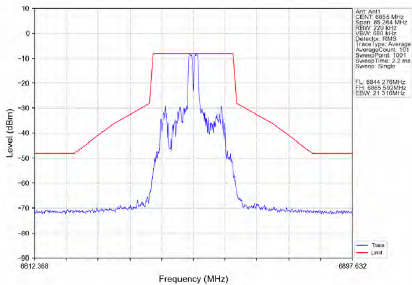
802.11ax(HE20)_HCH_6855MHz_RU26_Right_Ant1_NTNV
