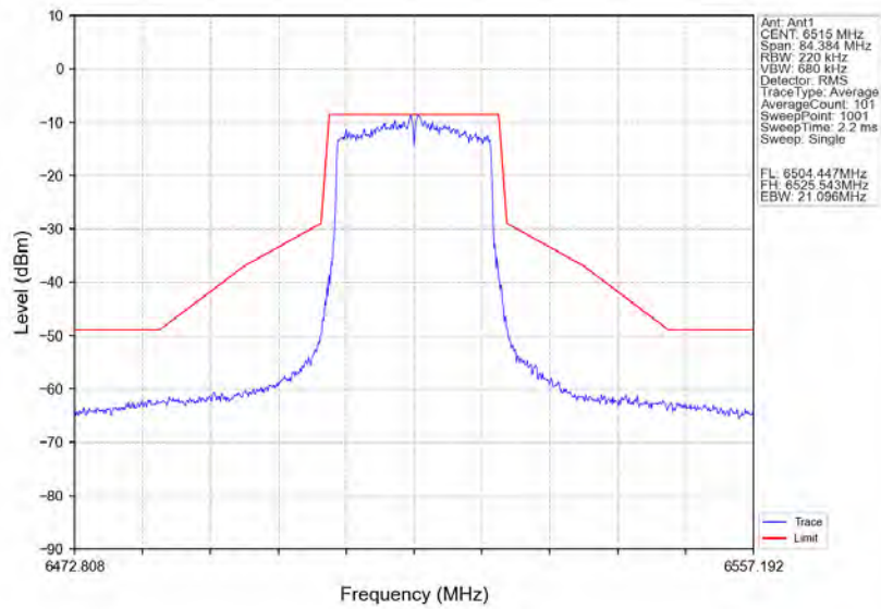
802.11ax(HE20)_HCH_6515MHz_RU242_Ant1_NTNV
