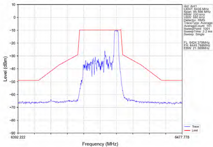
802.11ax(HE20)_LCH_6435MHz_RU26_Right_Ant1_NTNV
