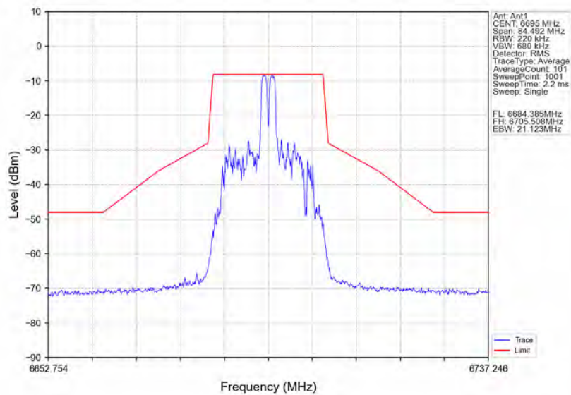
802.11ax(HE20)_MCH_6695MHz_RU26_Right_Ant1_NTNV
