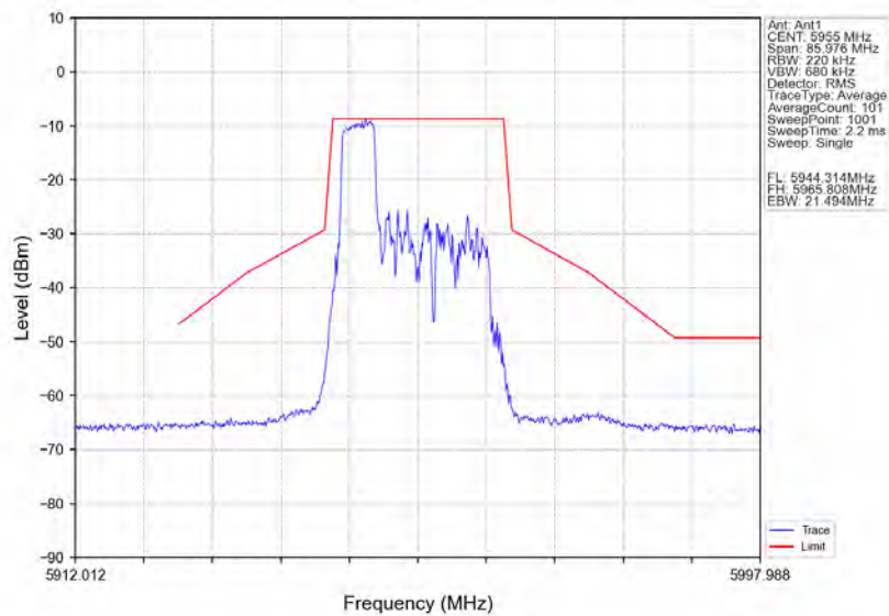
802.11ax(HE20)_LCH_5955MHz_RU52_Right_Ant1_NTNV
