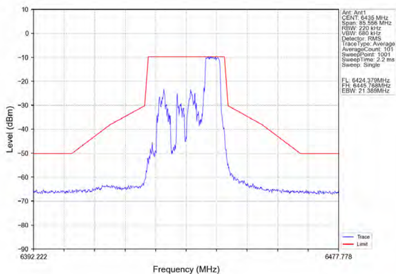
802.11ax(HE20)_LCH_6435MHz_RU52_Right_Ant1_NTNV
