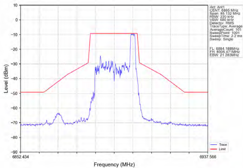
802.11ax(HE20)_LCH_6895MHz_RU26_Right_Ant1_NTNV
