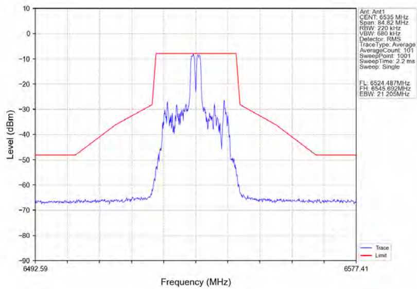
802.11ax(HE20)_LCH_6535MHz_RU26_Right_Ant1_NTNV
