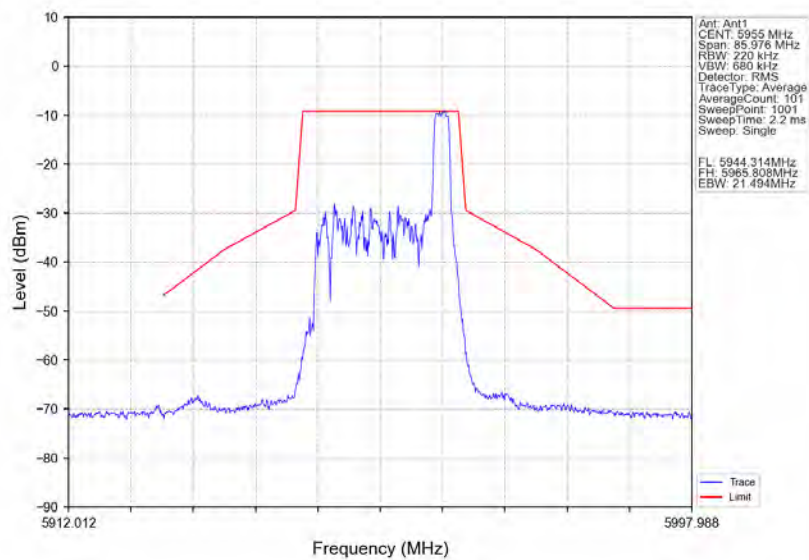
802.11ax(HE20)_LCH_5955MHz_RU26_Right_Ant1_NTNV
