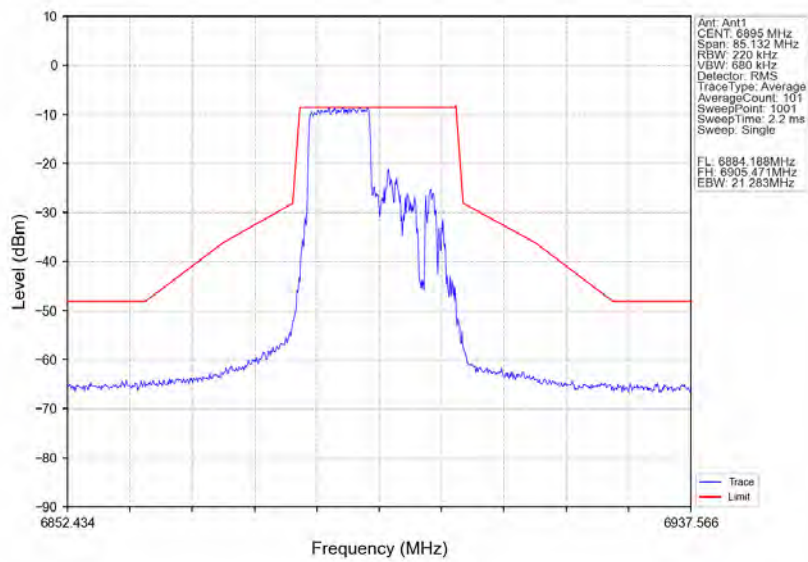
802.11ax(HE20)_LCH_6895MHz_RU106_Right_Ant1_NTNV
