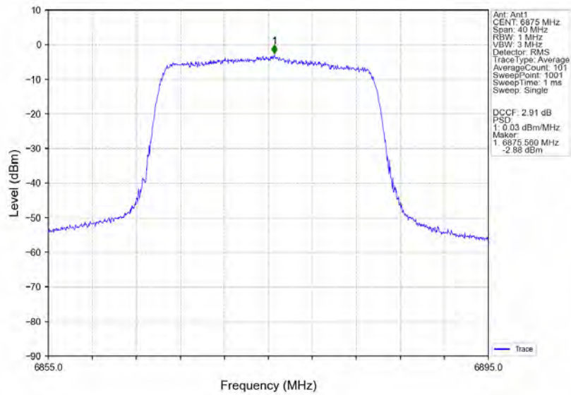
802.11ax(HE20)_HCH_6875MHz_RU242_Ant1_NTNV
