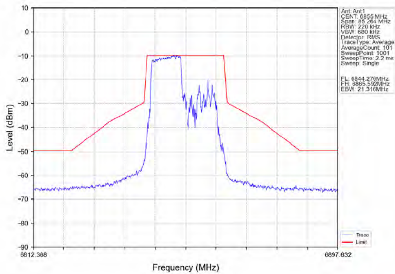
802.11ax(HE20)_HCH_6855MHz_RU106_Right_Ant1_NTNV
