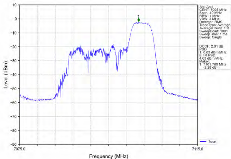
802.11ax(HE20) HCH_7095MHz_RU52_Right_Ant1_NTNV
