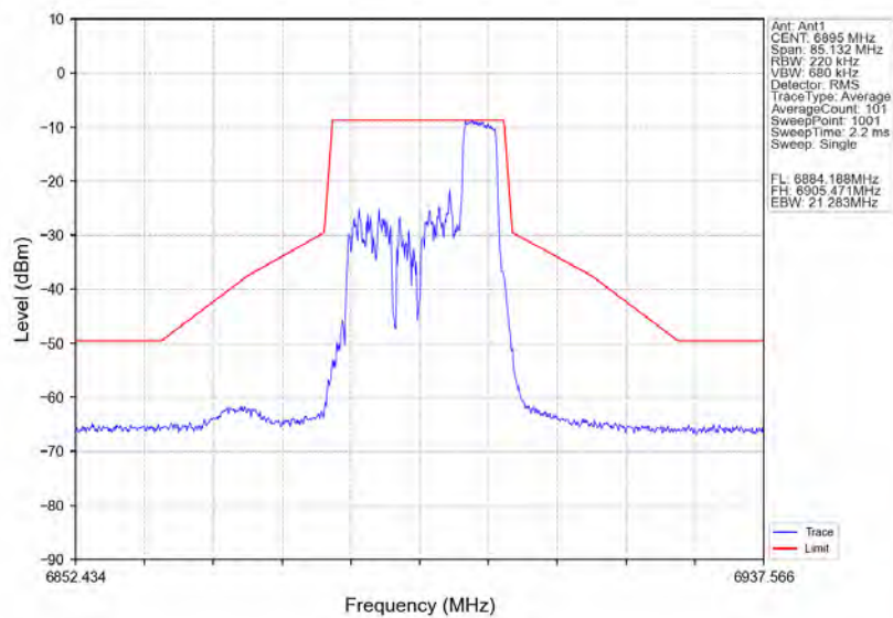
802.11ax(HE20)_LCH_6895MHz_RU52_Right_Ant1_NTNV
