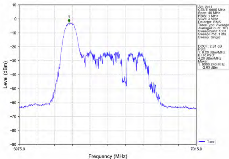
802.11ax(HE20)_MCH_6995MHz_RU26_Left_Ant1_NTNV
