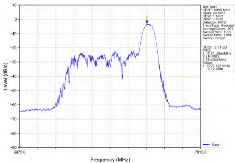
802.11ax(HE20)_MCH_6995MHz_RU26_Right_Ant1_NTNV
