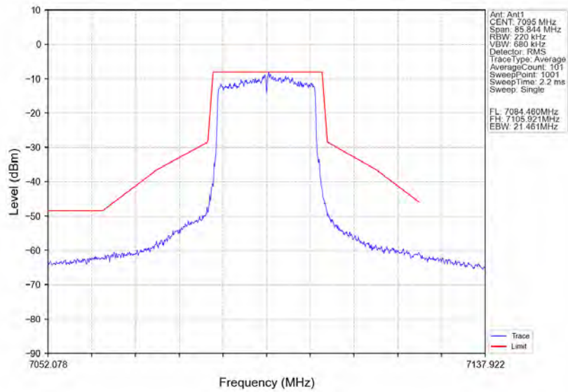
802.11ax(HE20)_HCH_7095MHz_RU242_Ant1_NTNV
