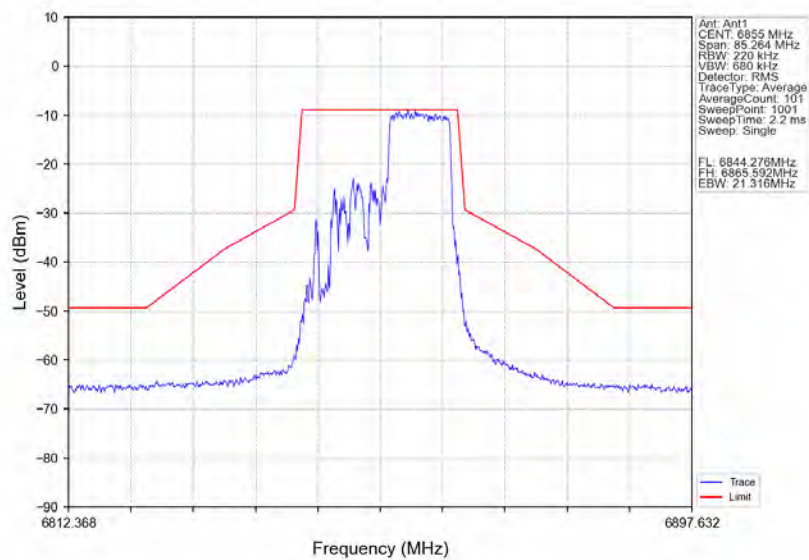
802.11ax(HE20)_HCH_6855MHz_RU106_Right_Ant1_NTNV
