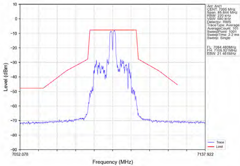
802.11ax(HE20)_HCH_7095MHz_RU26_Right_Ant1_NTNV
