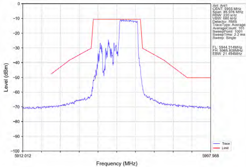
802.11ax(HE20)_LCH_5955MHz_RU106_Right_Ant1_NTNV
