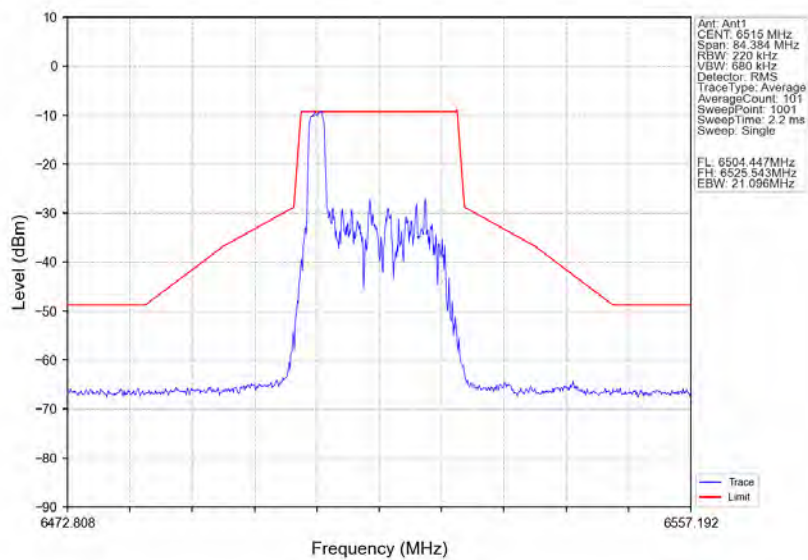
802.11ax(HE20)_HCH_6515MHz_RU26_Left_Ant1_NTNV
