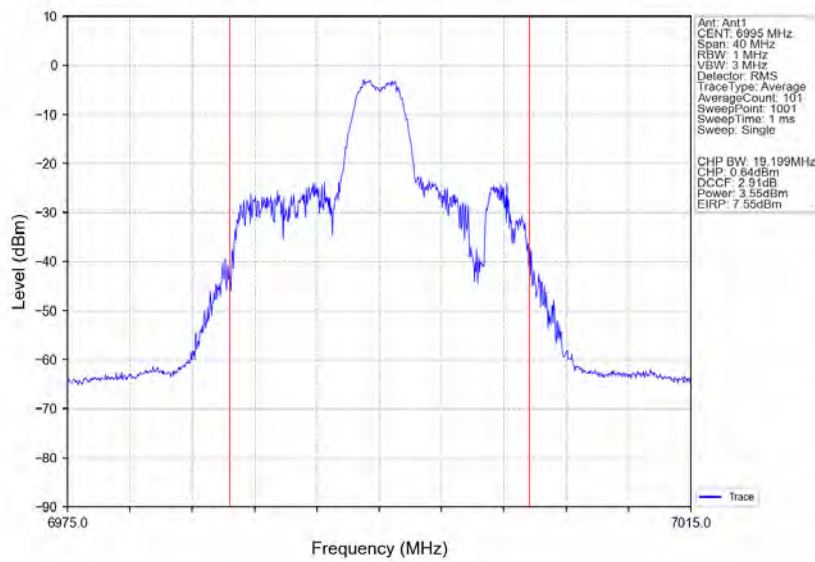
802.11ax(HE20)_MCH_6995MHz_RU26_Right_Ant1_NTNV
