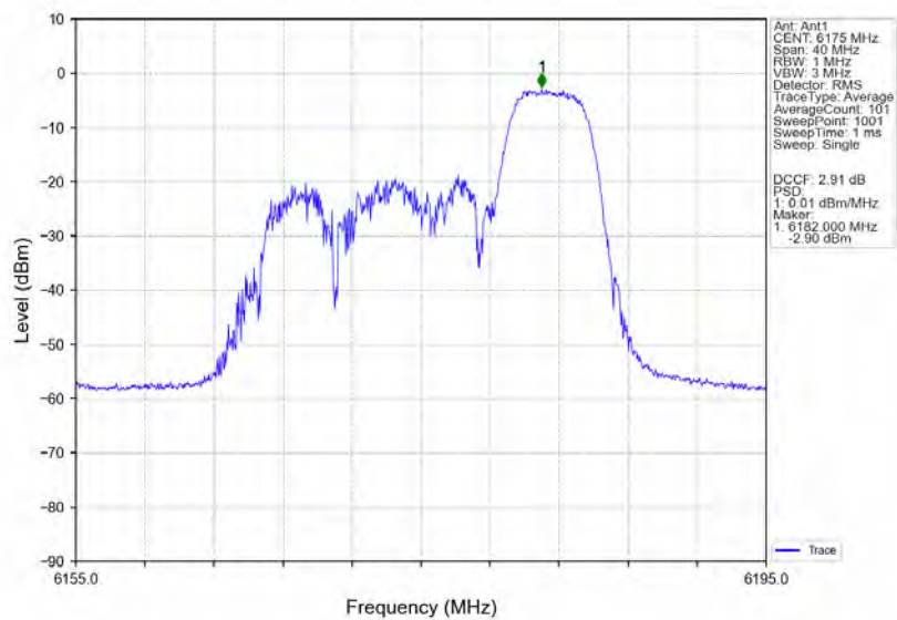
802.11ax(HE20)_MCH_6175MHz_RU52_Right_Ant1_NTNV
