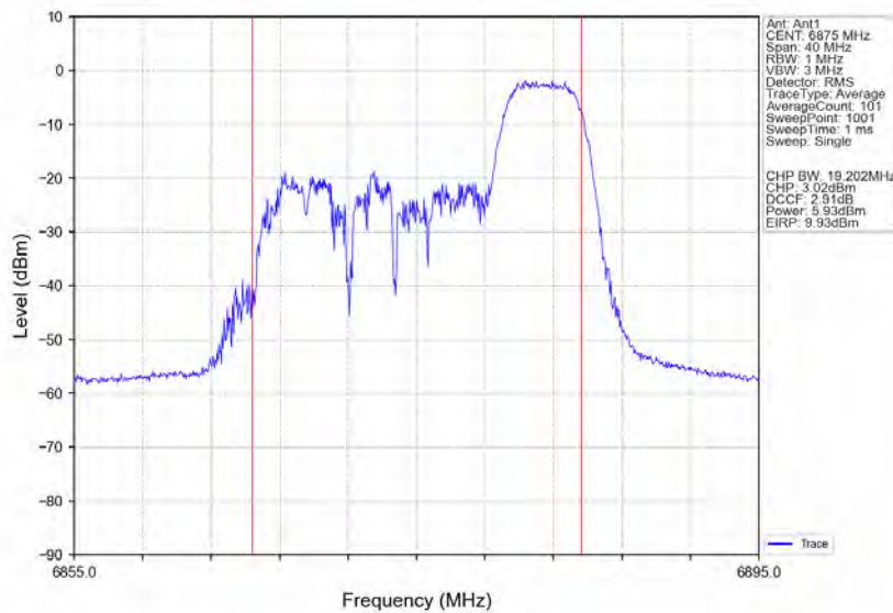
802.11ax(HE20) HCH_6875MHz_RU52_Right_Ant1_NTNV
