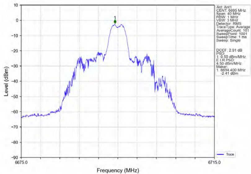
802.11ax(HE20)_MCH_6695MHz_RU26_Right_Ant1_NTNV
