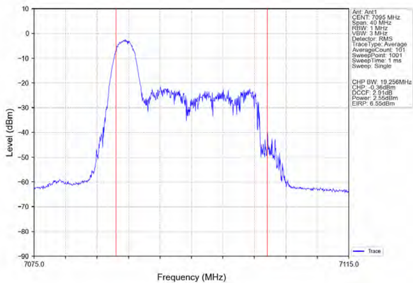
802.11ax(HE20)_HCH_7095MHz_RU26_Left_Ant1_NTNV
