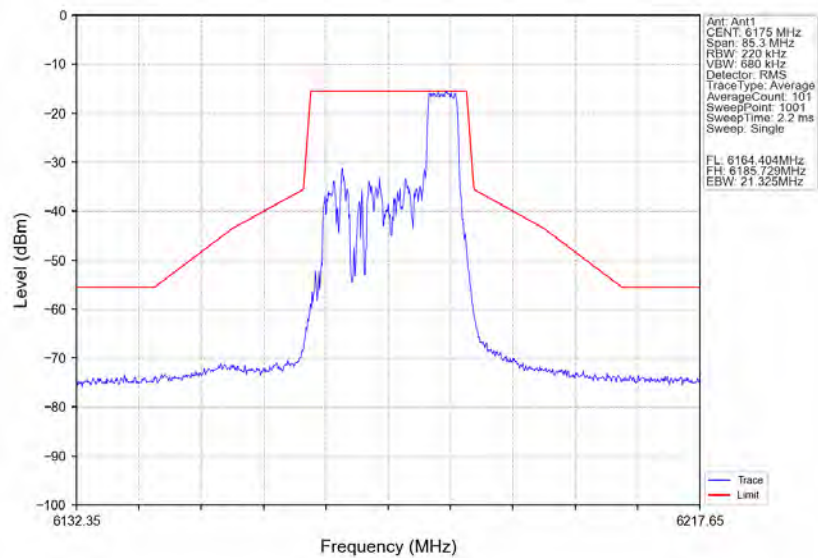
802.11ax(HE20)_MCH_6175MHz_RU52_Right_Ant1_NTNV
