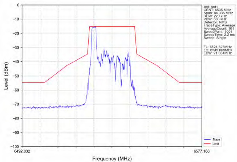
802.11ax(HE20)_LCH_6535MHz_RU26_Left_Ant1_NTNV
