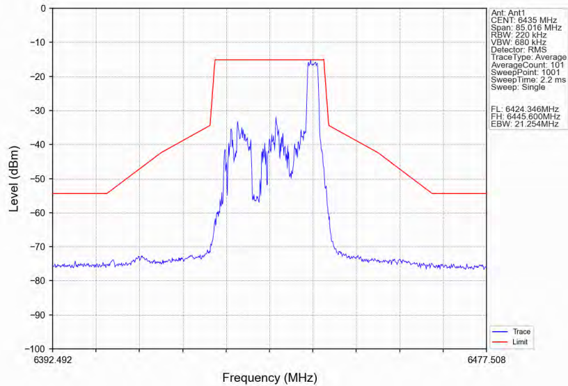
802.11ax(HE20)_LCH_6435MHz_RU26_Right_Ant1_NTNV
