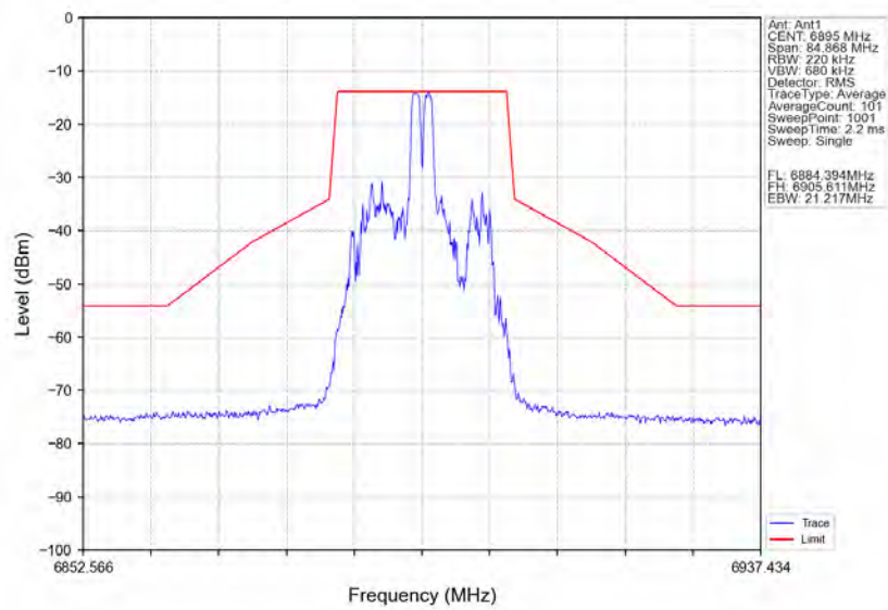
802.11ax(HE20)_LCH_6895MHz_RU26_Right_Ant1_NTNV
