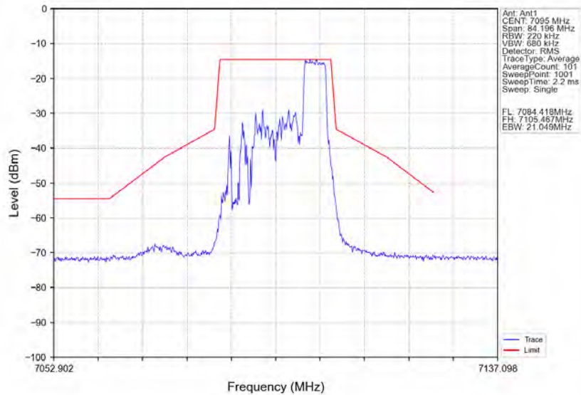
802.11ax(HE20) HCH_7095MHz_RU52_Right_Ant1_NTNV
