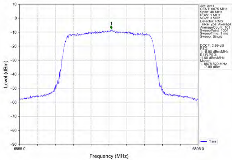
802.11ax(HE20)_HCH_6875MHz_RU242_Ant1_NTNV
