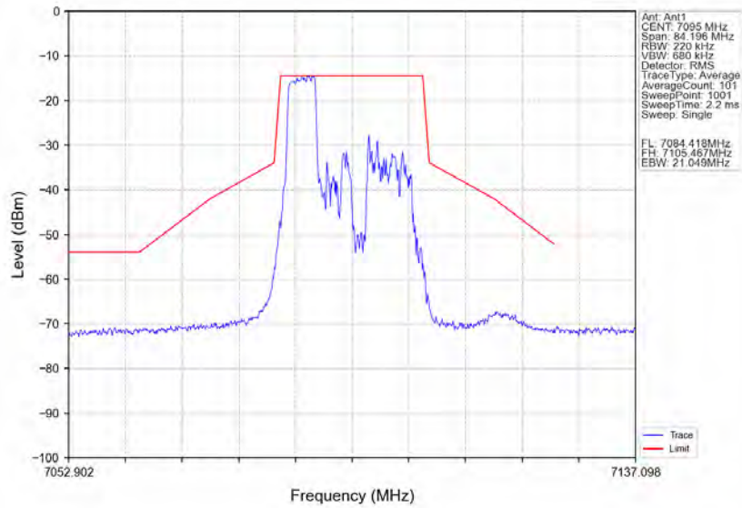
802.11ax(HE20) HCH_7095MHz_RU52_Right_Ant1_NTNV
