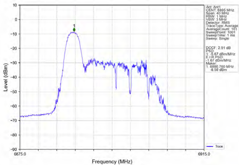
802.11ax(HE20)_LCH_6895MHz_RU26_Left_Ant1_NTNV
