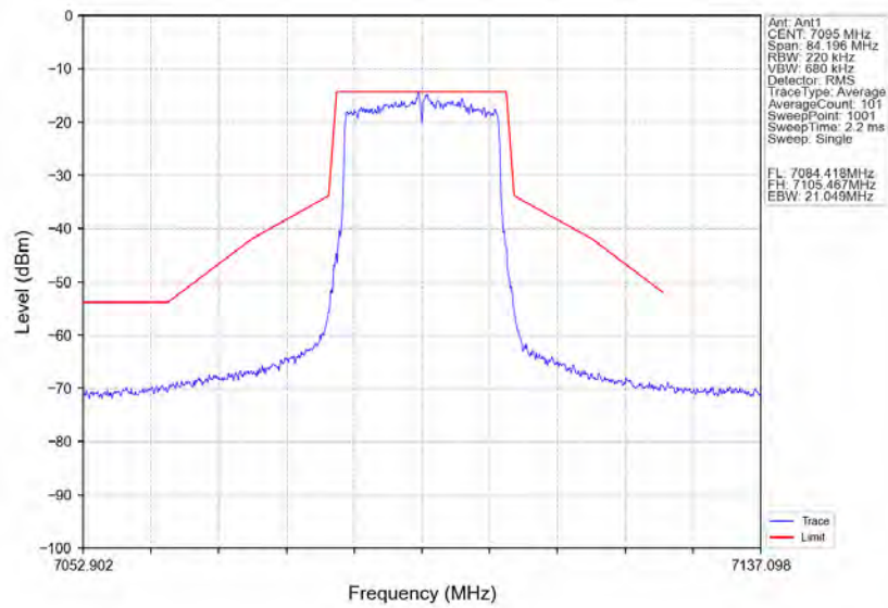
802.11ax(HE20)_HCH_7095MHz_RU242_Ant1_NTNV
