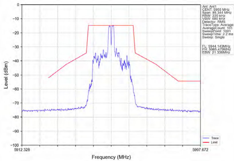
802.11ax(HE20)_LCH_5955MHz_RU26_Right_Ant1_NTNV
