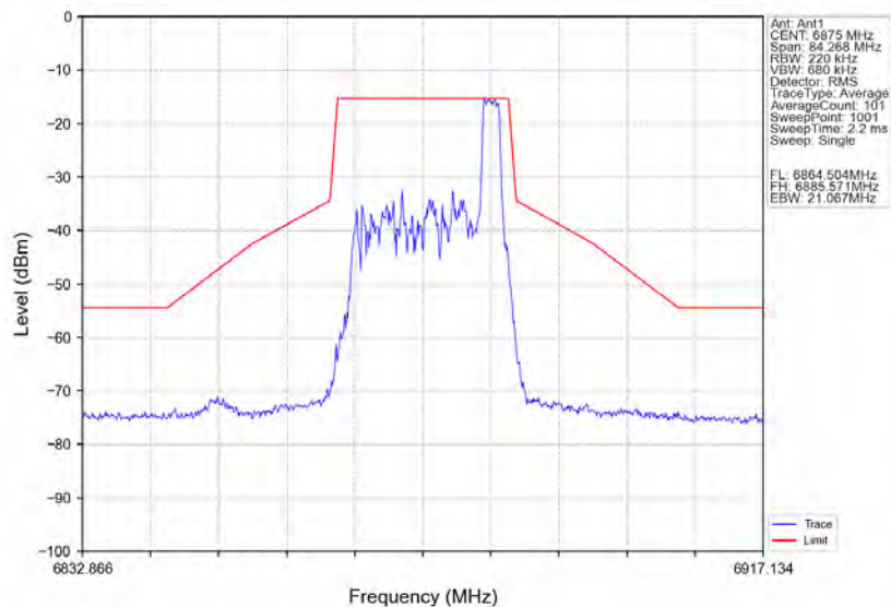
802.11ax(HE20)_HCH_6875MHz_RU26_Right_Ant1_NTNV
