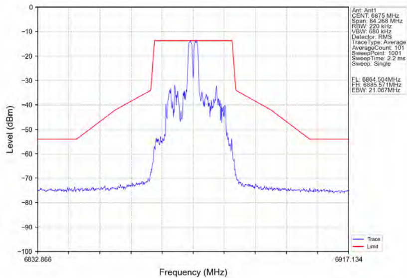
802.11ax(HE20)_HCH_6875MHz_RU26_Right_Ant1_NTNV
