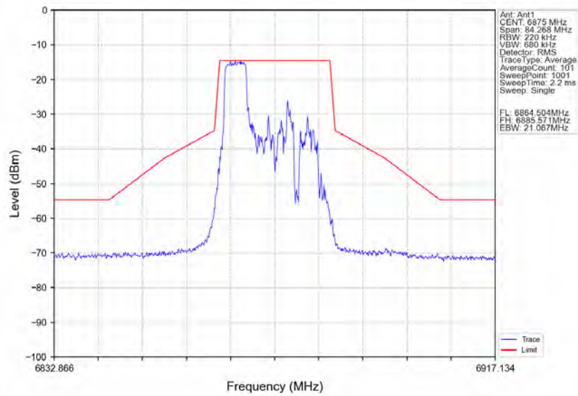
802.11ax(HE20) HCH_6875MHz_RU52_Right_Ant1_NTNV
