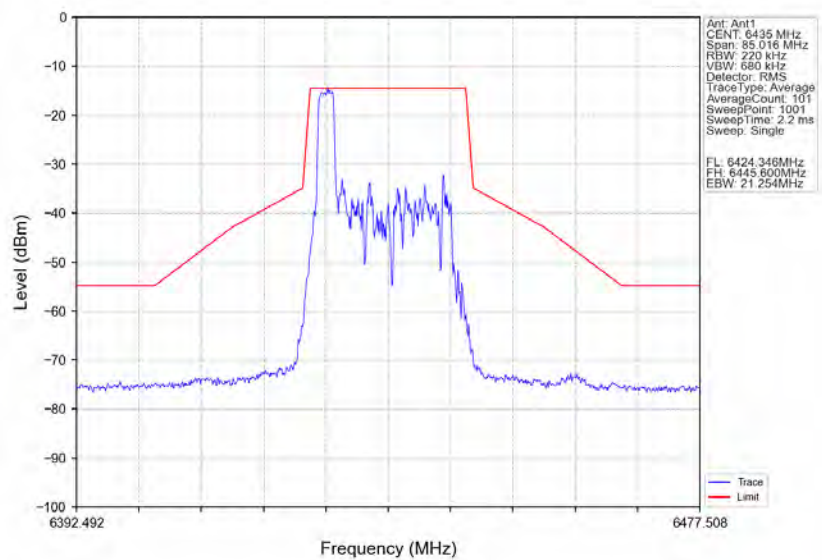
802.11ax(HE20)_LCH_6435MHz_RU26_Left_Ant1_NTNV
