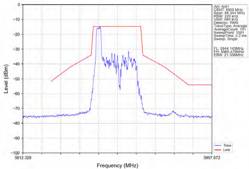
802.11ax(HE20)_LCH_5955MHz_RU26_Left_Ant1_NTNV
