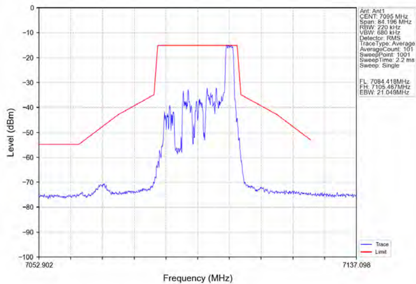
802.11ax(HE20) HCH_7095MHz_RU26_Right_Ant1_NTNV
