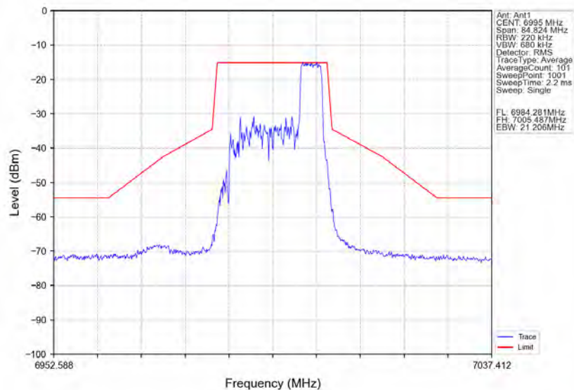
802.11ax(HE20)_MCH_6995MHz_RU52_Right_Ant1_NTNV
