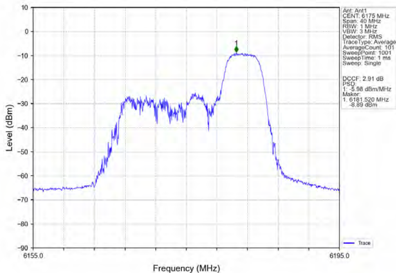
802.11ax(HE20)_MCH_6175MHz_RU52_Right_Ant1_NTNV
