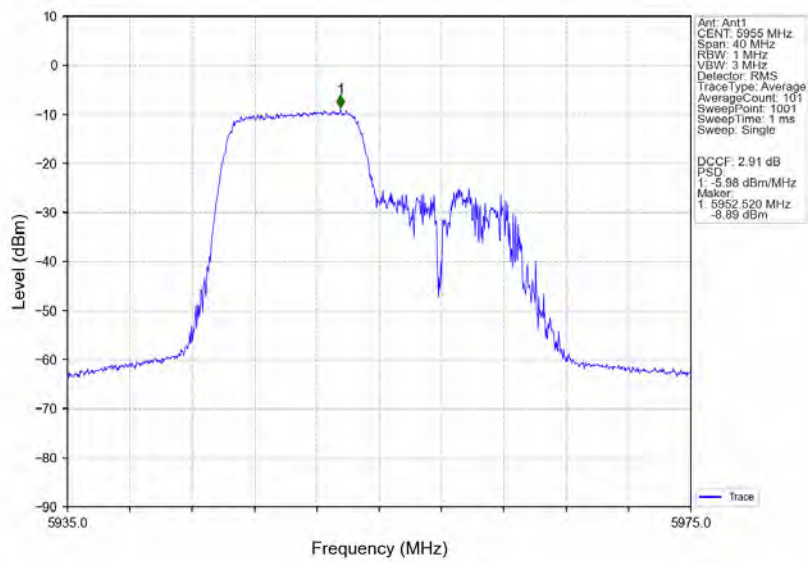
802.11ax(HE20)_LCH_5955MHz_RU106_Right_Ant1_NTNV
