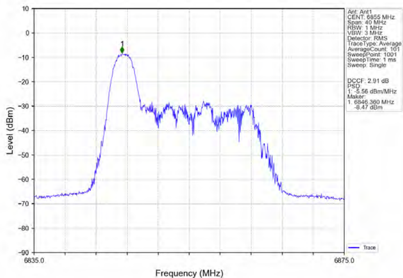
802.11ax(HE20)_HCH_6855MHz_RU26_Left_Ant1_NTNV
