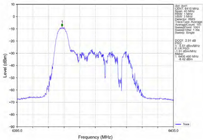
802.11ax(HE20)_HCH_6415MHz_RU26_Left_Ant1_NTNV
