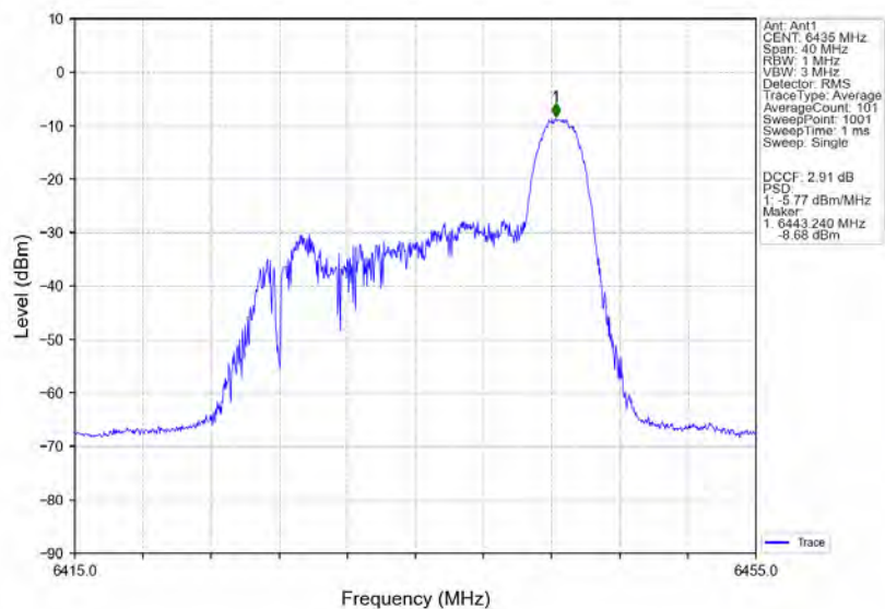
802.11ax(HE20)_LCH_6435MHz_RU26_Right_Ant1_NTNV
