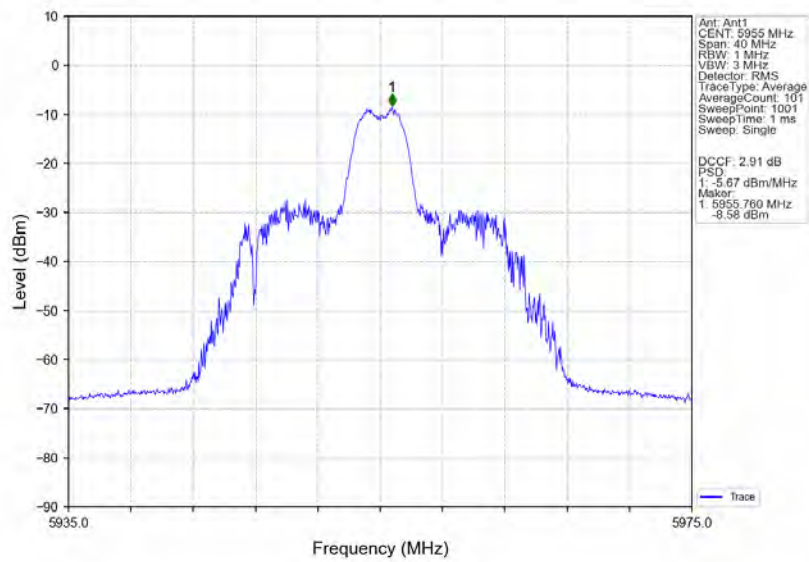
802.11ax(HE20)_LCH_5955MHz_RU26_Right_Ant1_NTNV
