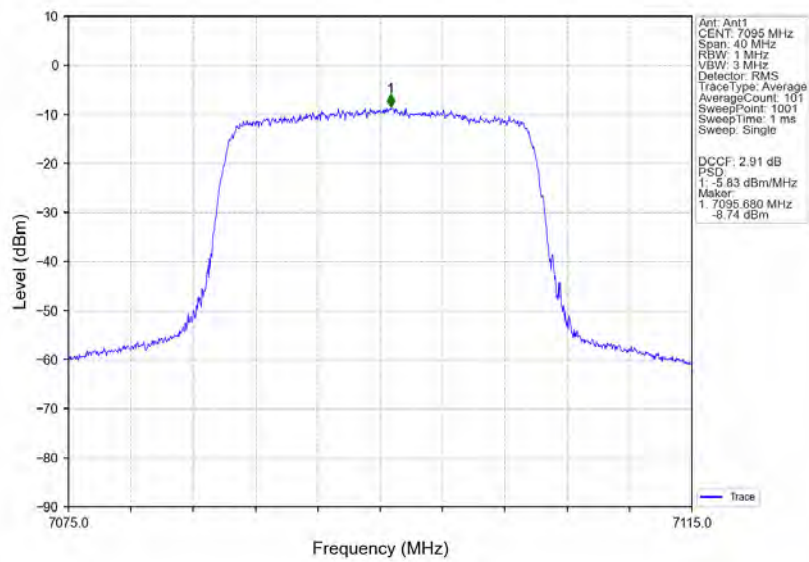
802.11ax(HE20)_HCH_7095MHz_RU242_Ant1_NTNV
