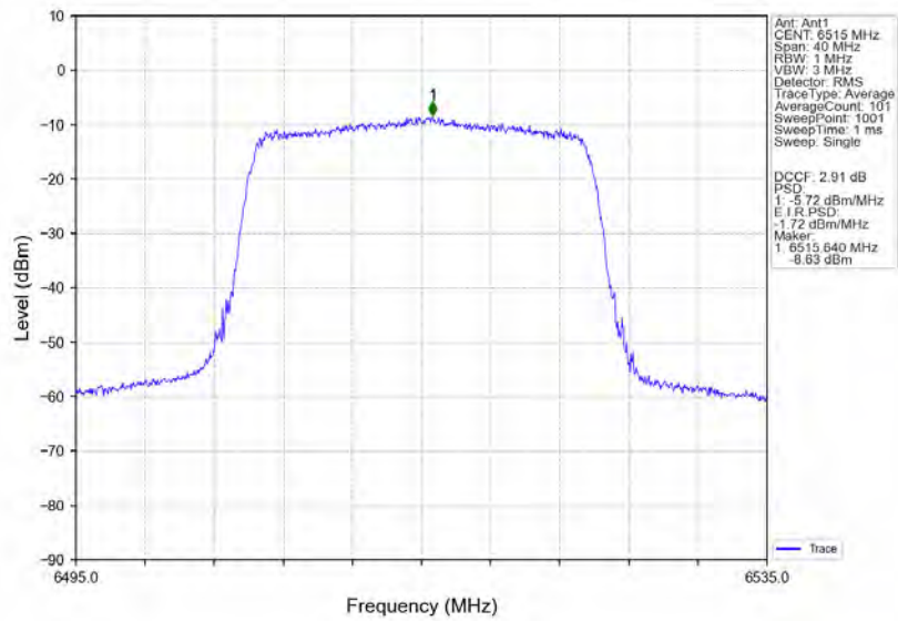
802.11ax(HE20)_HCH_6515MHz_RU242_Ant1_NTNV
