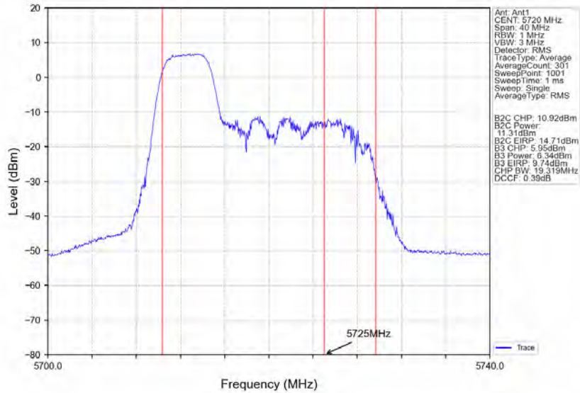
802.11ax(HE20)_HCH_5720MHz_RU106_Left_Ant1_NTNV
