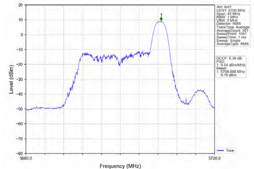
802.11ax(HE20)_HCH_5700MHz_RU26_Right_Ant1_NTNV
