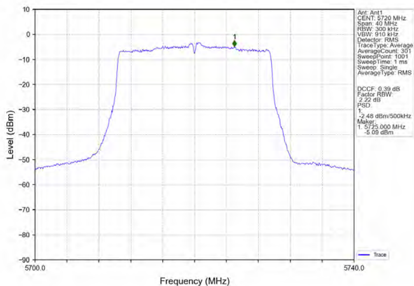
802.11ax(HE20)_HCH_5720MHz_RU242_Ant1_NTNV
