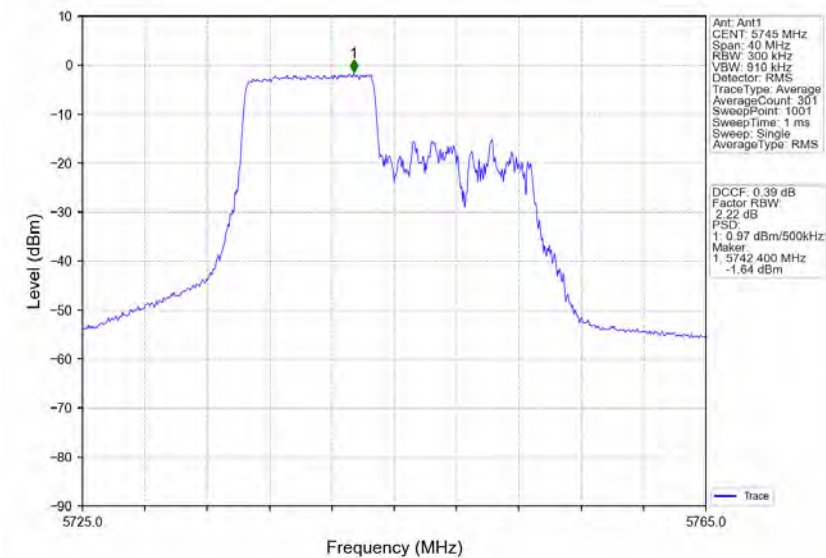
802.11ax(HE20)_LCH_5745MHz_RU242_Ant1_NTNV
