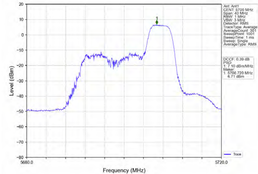
802.11ax(HE20)_HCH_5700MHz_RU52_Right_Ant1_NTNV
