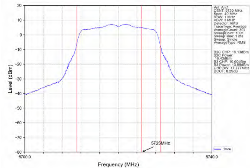
802.11a_HCH_5720MHz_Ant1_NTNV
