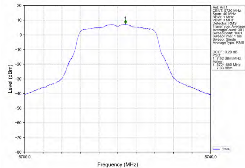
802.11a_HCH_5720MHz_Ant1_NTNV
