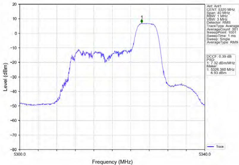
802.11ax(HE20)_HCH_5320MHz_RU106_Right_Ant1_NTNV
