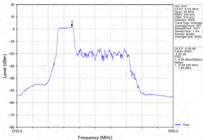
802.11ax(HE20)_LCH_5745MHz_RU52_Left_Ant1_NTNV
