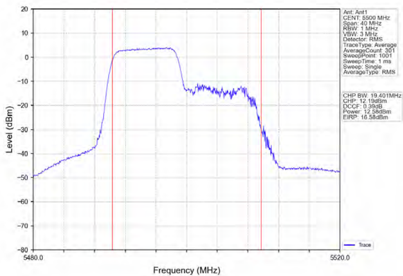
802.11ax(HE20)_LCH_5500MHz_RU106_Left_Ant1_NTNV
