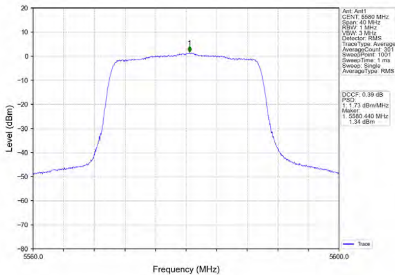
802.11ax(HE20)_MCH_5580MHz_RU242_Ant1_NTNV
