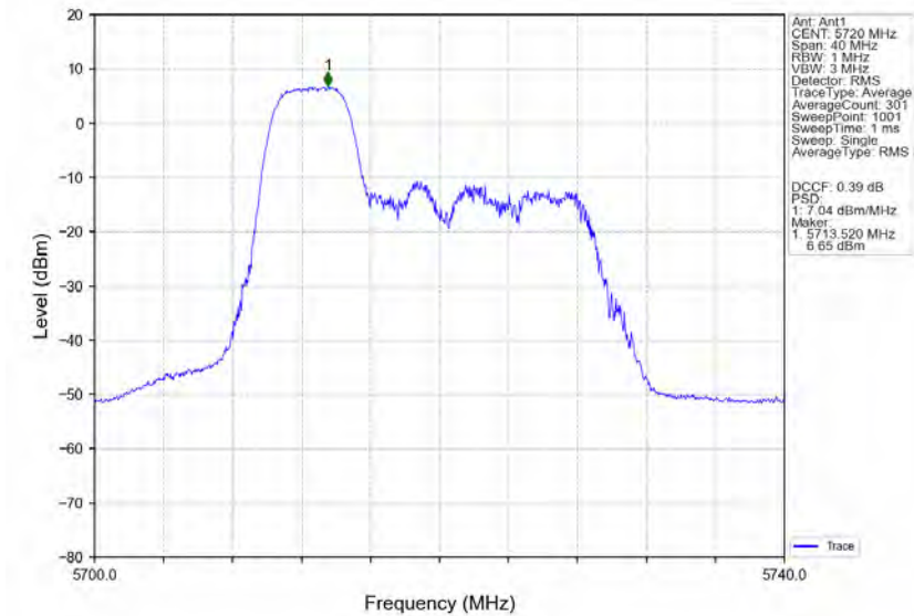
802.11ax(HE20)_HCH_5720MHz_RU52_Left_Ant1_NTNV
