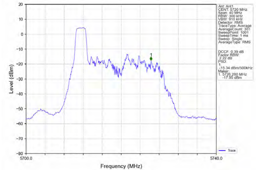
802.11ax(HE20)_HCH_5720MHz_RU52_Left_Ant1_NTNV
