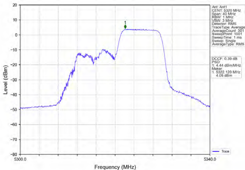
802.11ax(HE20)_HCH_5320MHz_RU106_Right_Ant1_NTNV
