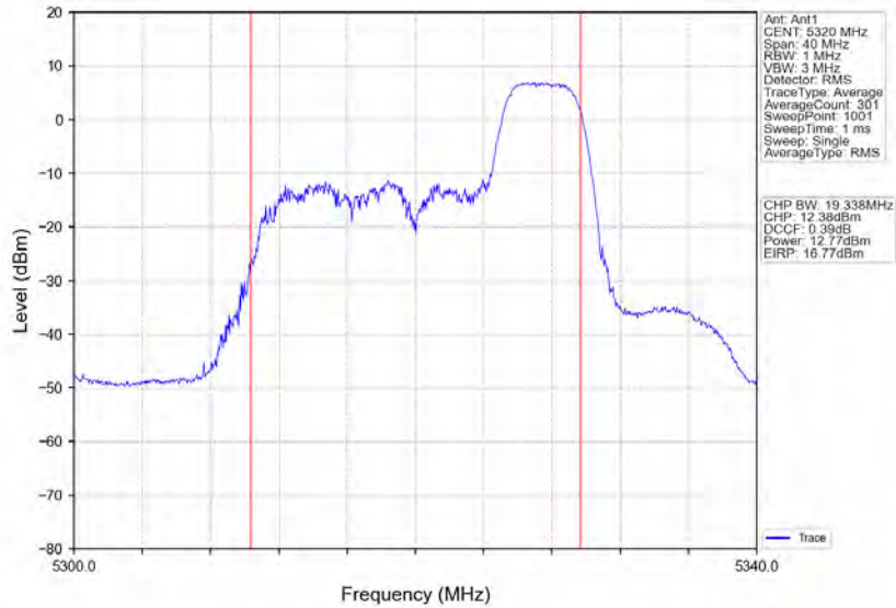
802.11ax(HE20)_HCH_5320MHz_RU106_Right_Ant1_NTNV
