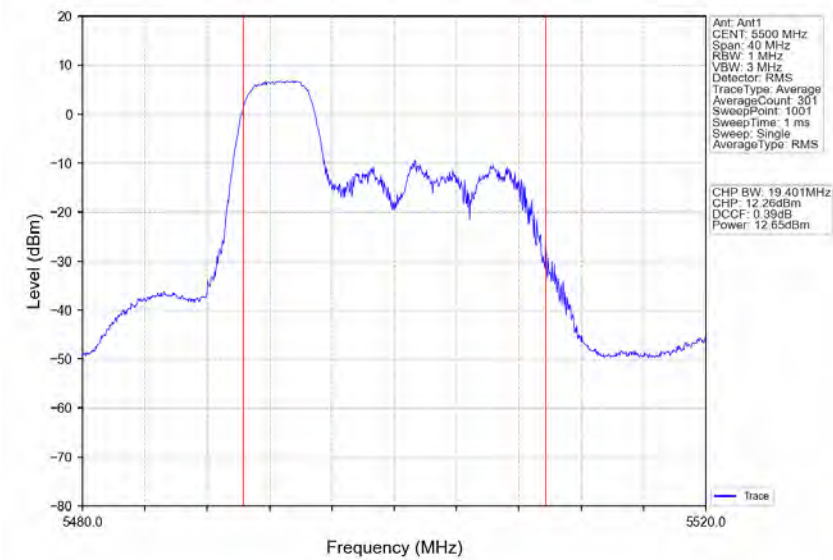
802.11ax(HE20)_LCH_5500MHz_RU106_Left_Ant1_NTNV
