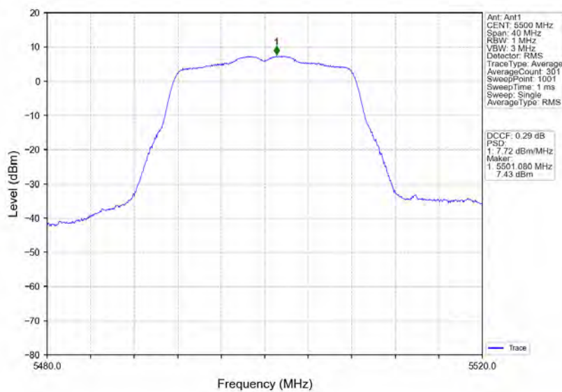
802.11a_LCH_5500MHz_Ant1_NTNV
