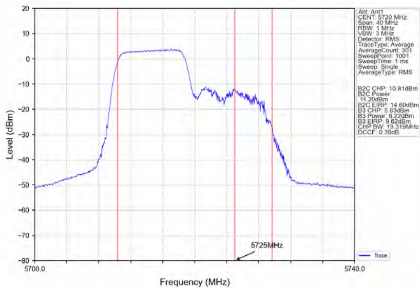
802.11ax(HE20)_HCH_5720MHz_RU106_Left_Ant1_NTNV
