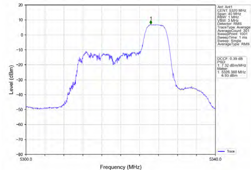
802.11ax(HE20)_HCH_5320MHz_RU52_Right_Ant1_NTNV
