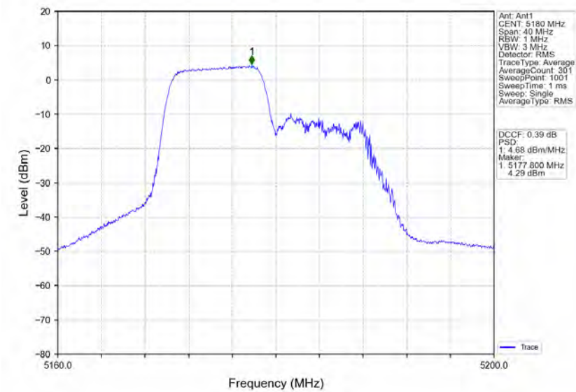
802.11ax(HE20)_LCH_5180MHz_RU242_Ant1_NTNV
