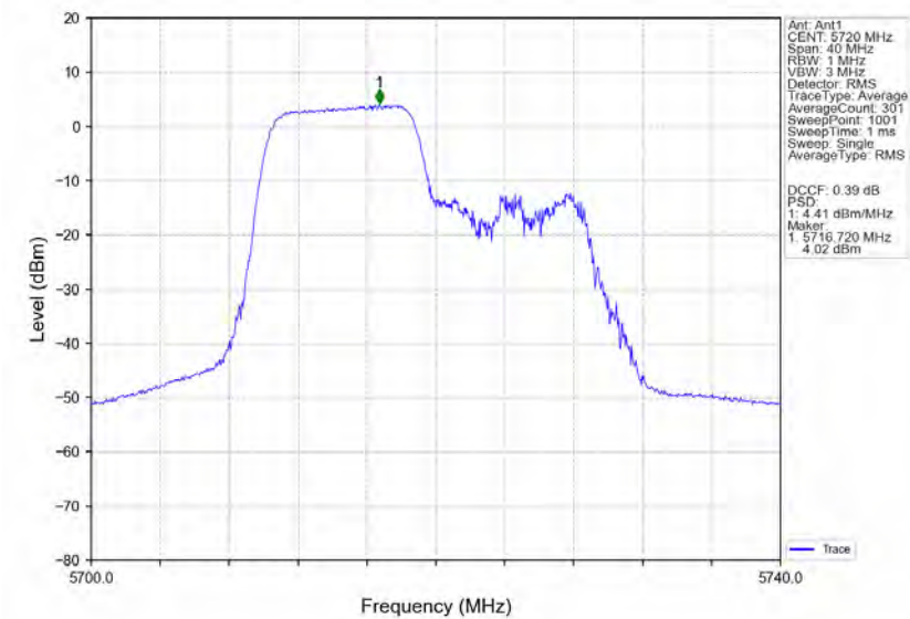
802.11ax(HE20)_HCH_5720MHz_RU106_Left_Ant1_NTNV
