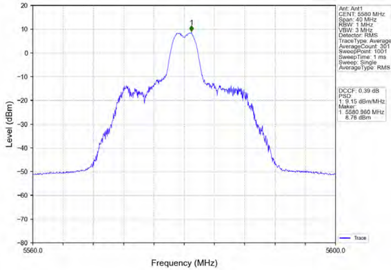
802.11ax(HE20)_MCH_5580MHz_RU242_Ant1_NTNV
