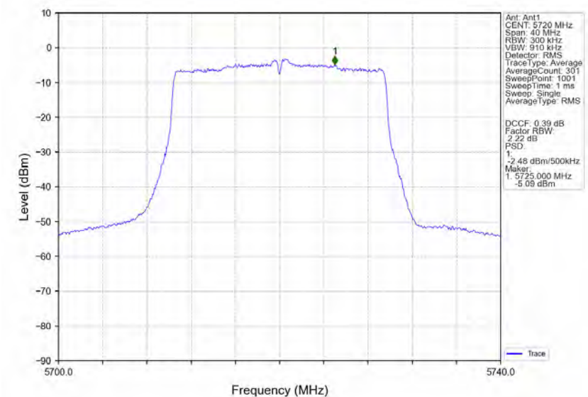
802.11ax(HE20)_HCH_5720MHz_RU242_Ant1_NTNV
