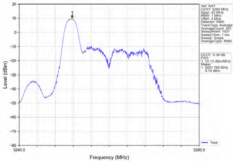
802.11ax(HE20)_LCH_5260MHz_RU52_Left_Ant1_NTNV
