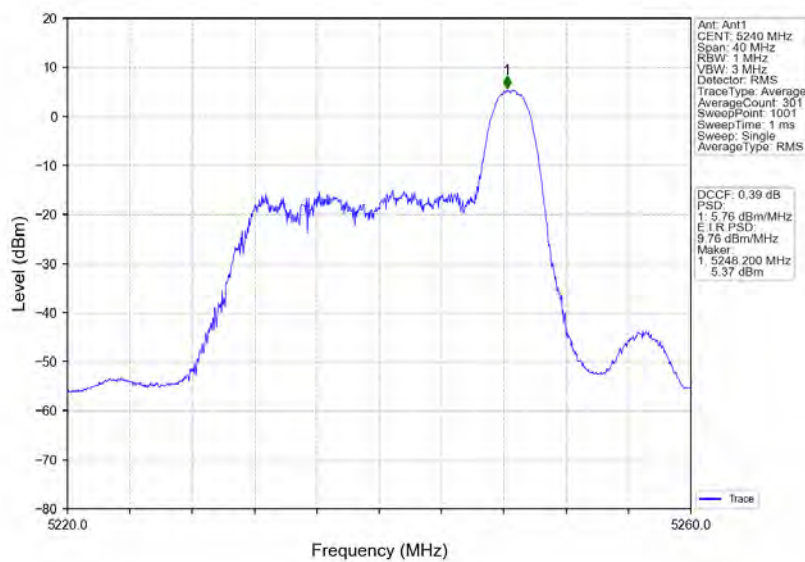
802.11ax(HE20)_HCH_5240MHz_RU26_Right_Ant1_NTNV
