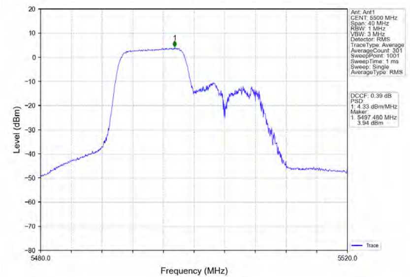
802.11ax(HE20)_LCH_5500MHz_RU242_Ant1_NTNV
