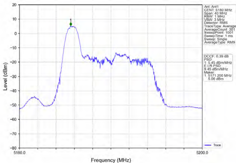
802.11ax(HE20)_LCH_5180MHz_RU26_Left_Ant1_NTNV
