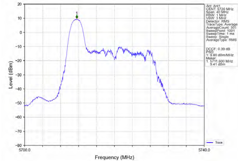
802.11ax(HE20)_HCH_5720MHz_RU52_Left_Ant1_NTNV
