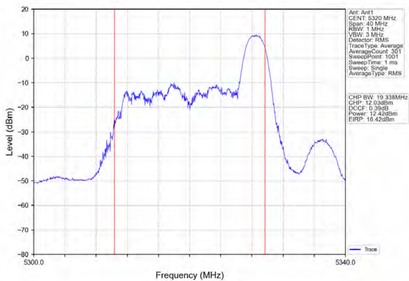
802.11ax(HE20)_HCH_5320MHz_RU26_Right_Ant1_NTNV
