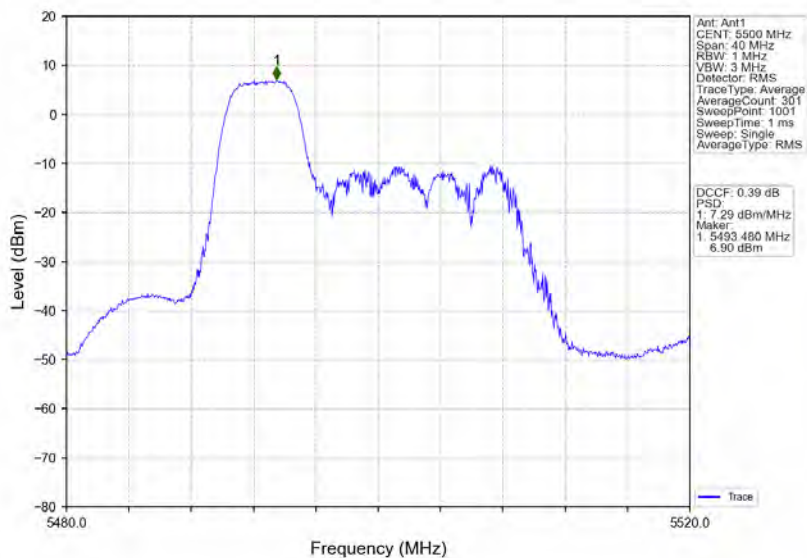
802.11ax(HE20)_LCH_5500MHz_RU52_Left_Ant1_NTNV
