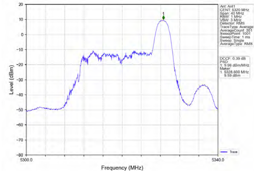
802.11ax(HE20)_HCH_5320MHz_RU52_Right_Ant1_NTNV
