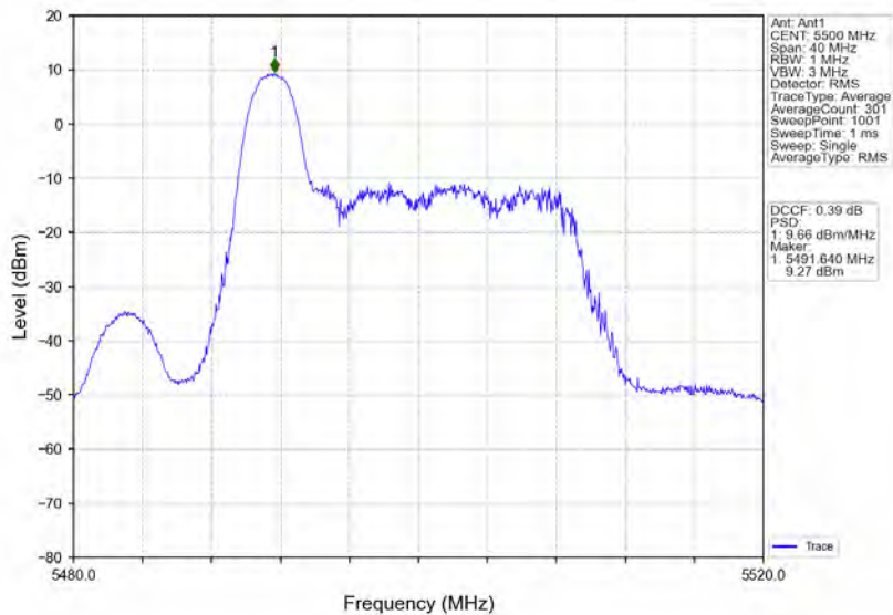
802.11ax(HE20)_LCH_5500MHz_RU52_Left_Ant1_NTNV
