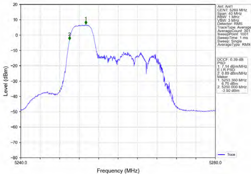
802.11ax(HE20)_LCH_5260MHz_RU106_Left_Ant1_NTNV
