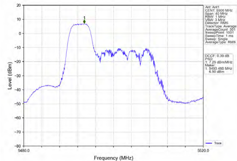
802.11ax(HE20)_LCH_5500MHz_RU106_Left_Ant1_NTNV
