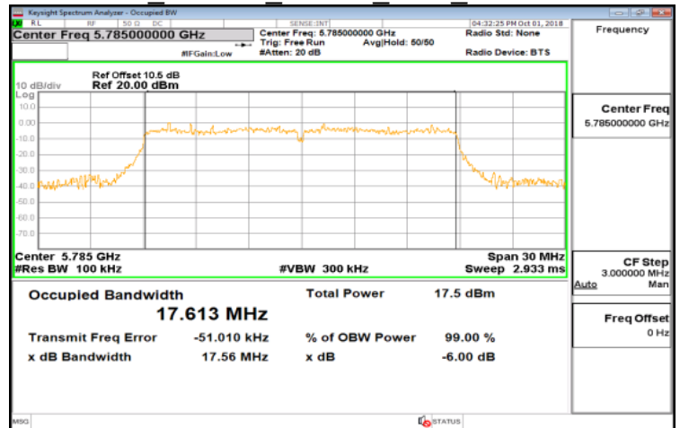
FCC 802.11n 20MHz Main 5785MHz
