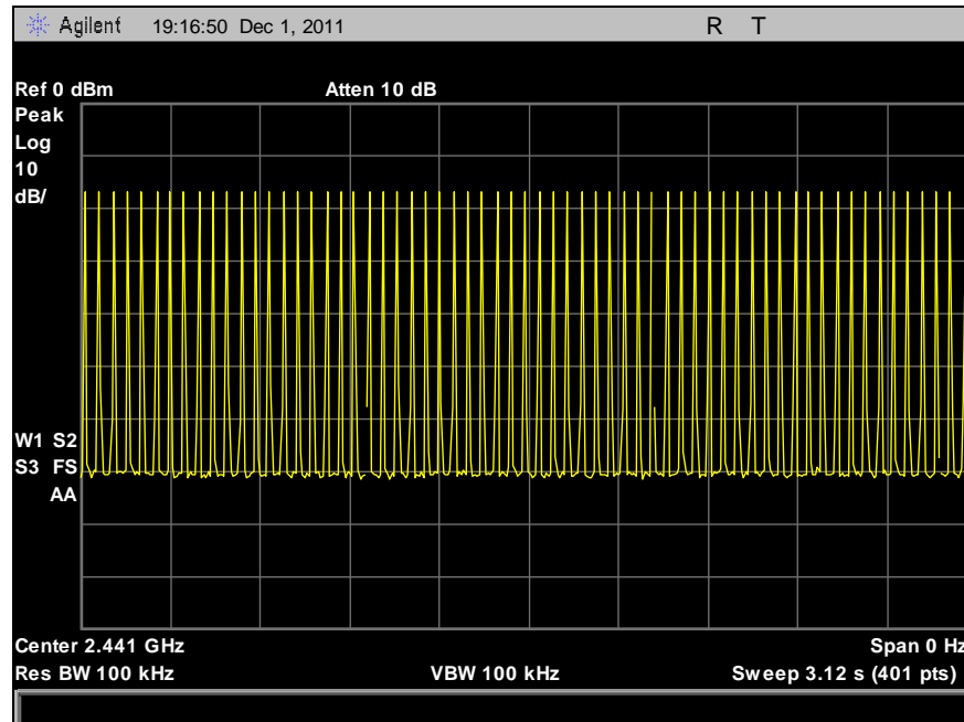
Plot 11. DH 1 Burst (63)
