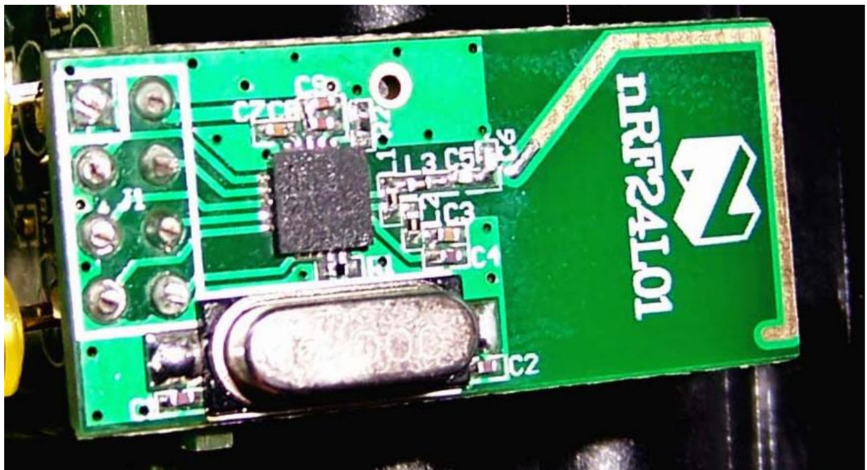
RF_Remote_Front
