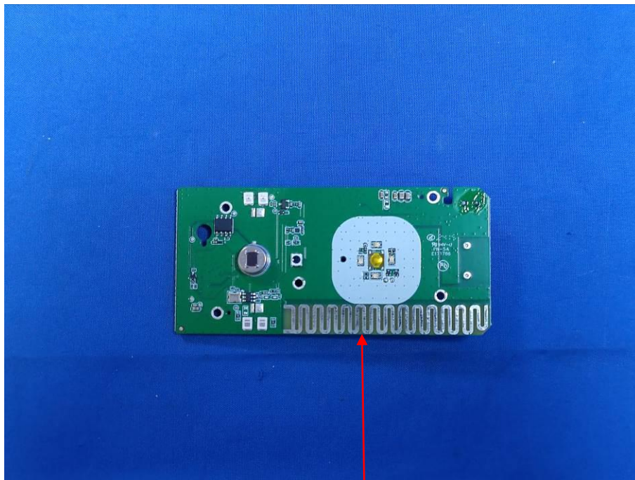
433M antenna
