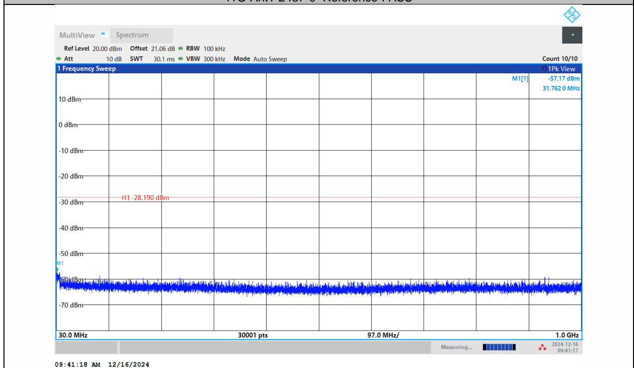
11G-Ant1-2437-30~1000-PASS
