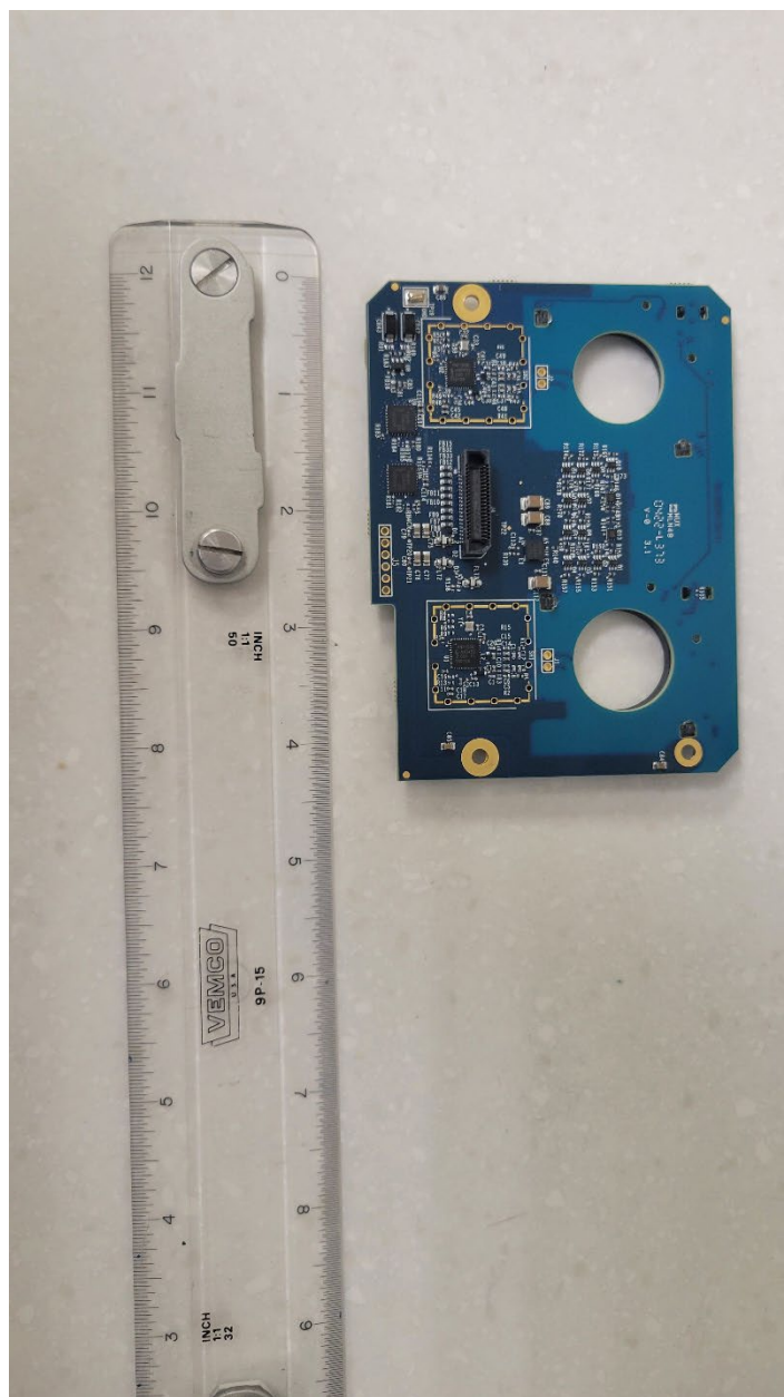
NGTL PCB side 2
