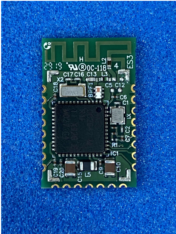
Top side(No Shield case)
