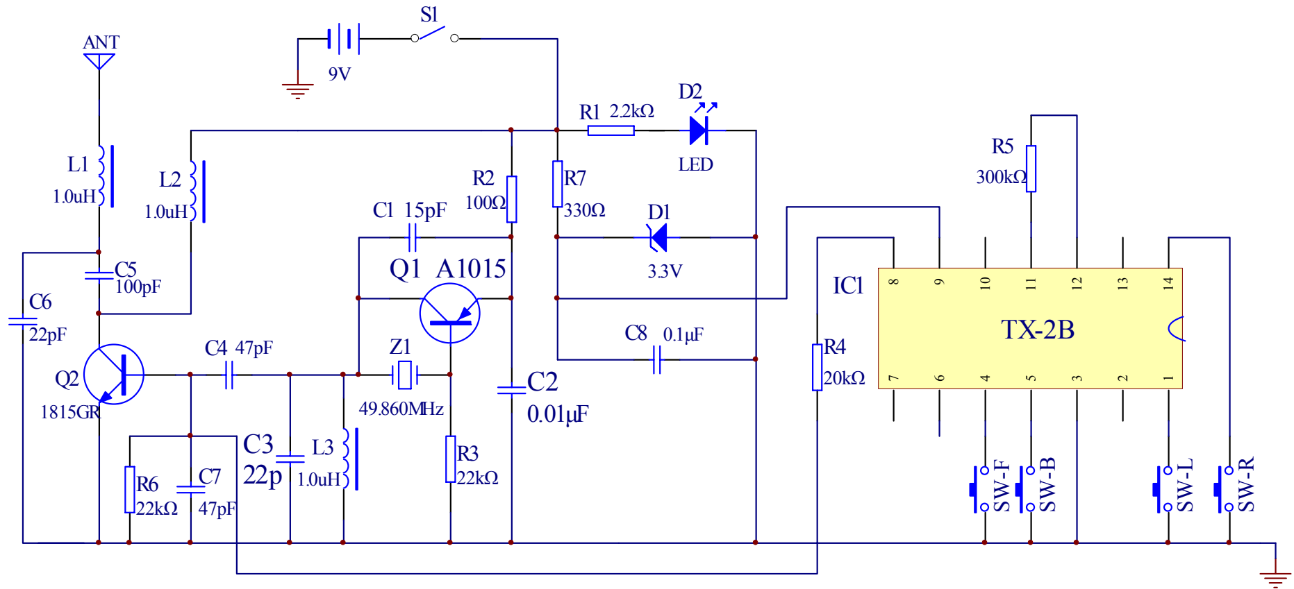
ZHT-061T-ZJ 49MHz 发射电路原理图
