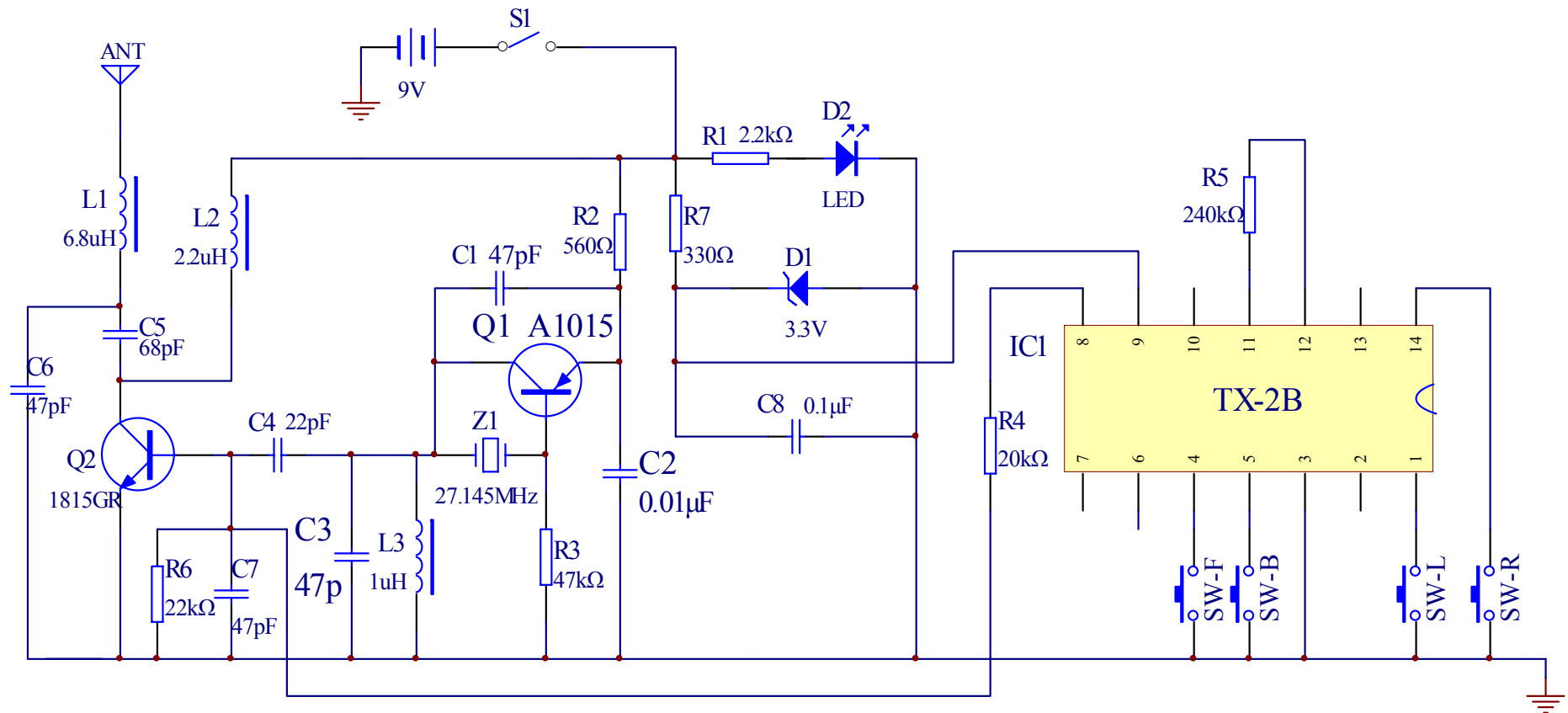
ZHT-061T-ZJ 27MHz发射电路原理图
