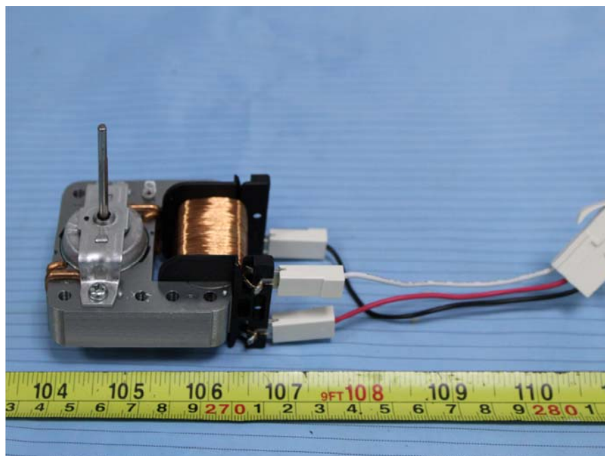
EUT – Fan Motor View
