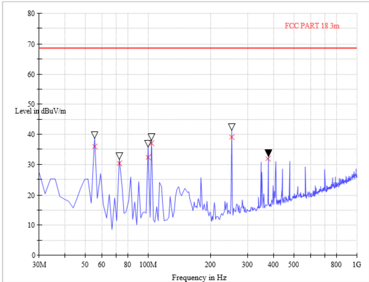
(Plot A: Test Antenna Horizontal 30M - 1G)
