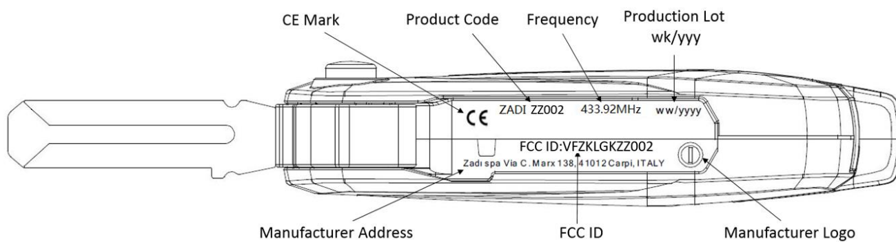
Label lay-out
