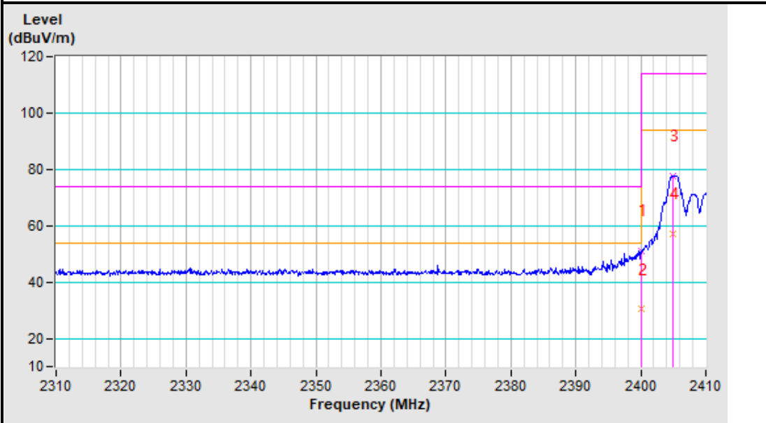
2405MHz Vertical
