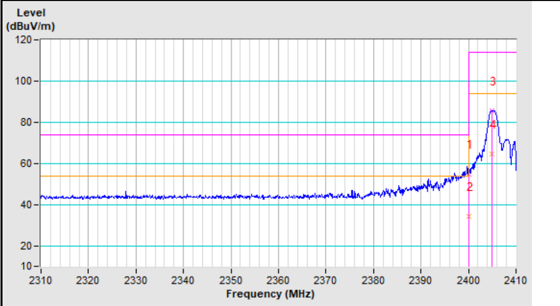
2405MHz Vertical
