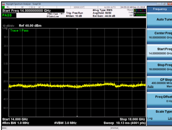
LTE10 Top+NB IoT GB (Upper) 14000MHz-18000MHz
