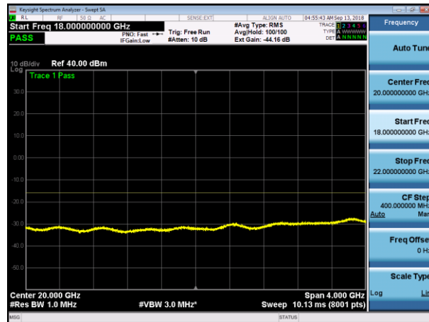
LTE10 Top+NB IoT GB (Upper) 18000MHz-22000MHz
