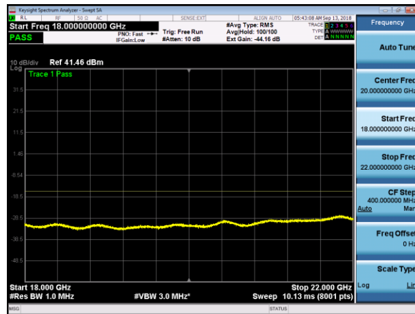
LTE15 Mid+NB IoT GB (Upper) 18000MHz-22000MHz
