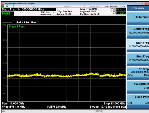
LTE15 Mid+NB IoT GB (Upper) 14000MHz-18000MHz
