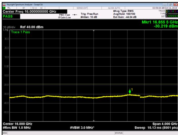
Band 66, LTE10, M, Upper, 14GHz-18GHz
