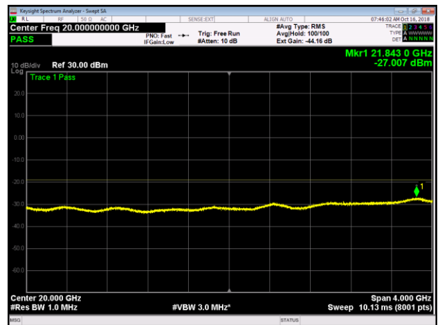
Band 66, LTE10, B, Upper, 18GHz-22GHz
