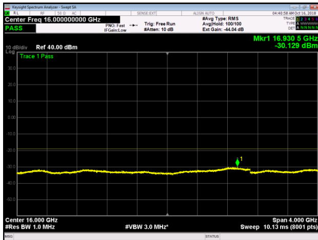
Band 25, LTE10, B, Upper, 14GHz-18GHz
