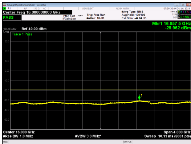
Band 66, LTE10, T, Upper, 14GHz-18GHz
