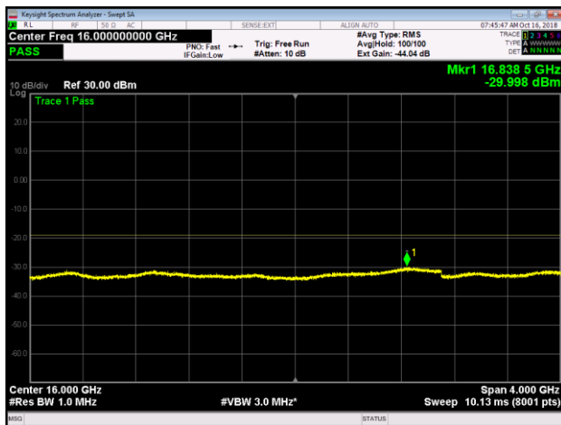
Band 66, LTE10, B, Upper, 14GHz-18GHz
