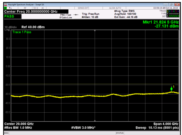
Band 66, LTE10, M, Upper, 18GHz-22GHz
