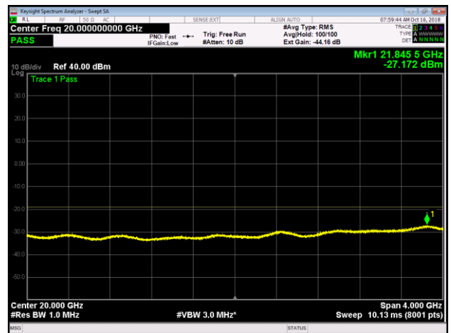
Band 66, LTE10, T, Upper, 18GHz-22GHz
