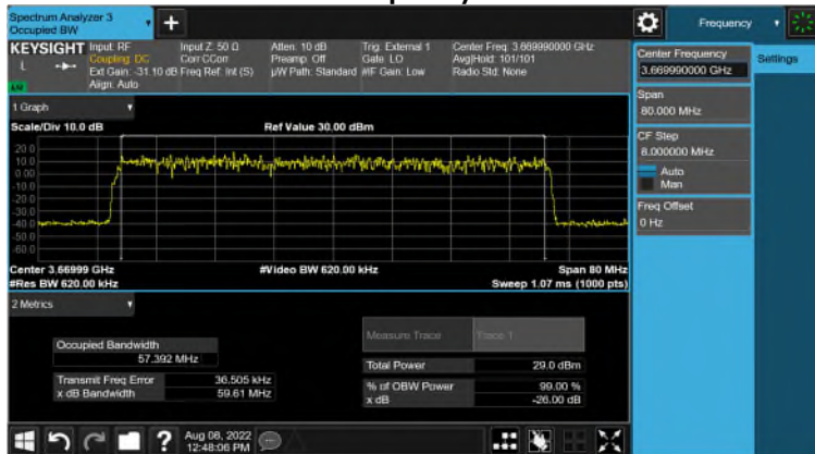
60MHz BW, TM3.1a Channel Frequency 3670MHz
