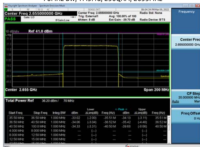
70MHz BW, TM3.1a, 256QAM, 2655MHz
