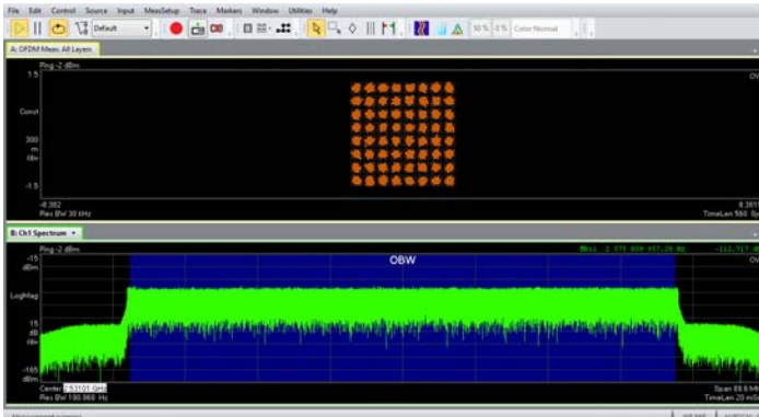
TM3.1 / 64QAM / 2531MHz
