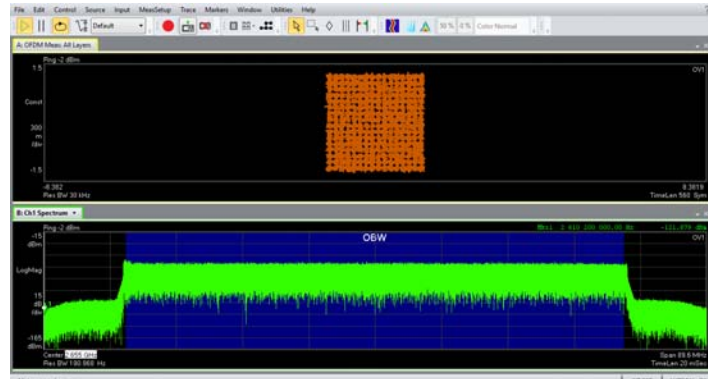
TM3.1a / 256QAM / 2655MHz
