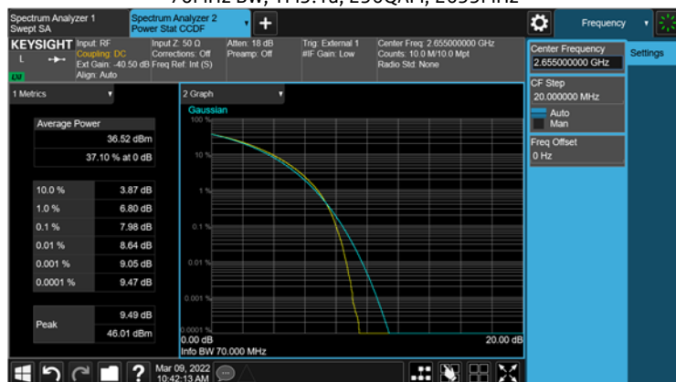
70MHz BW, TM3.1a, 256QAM, 2655MHz
