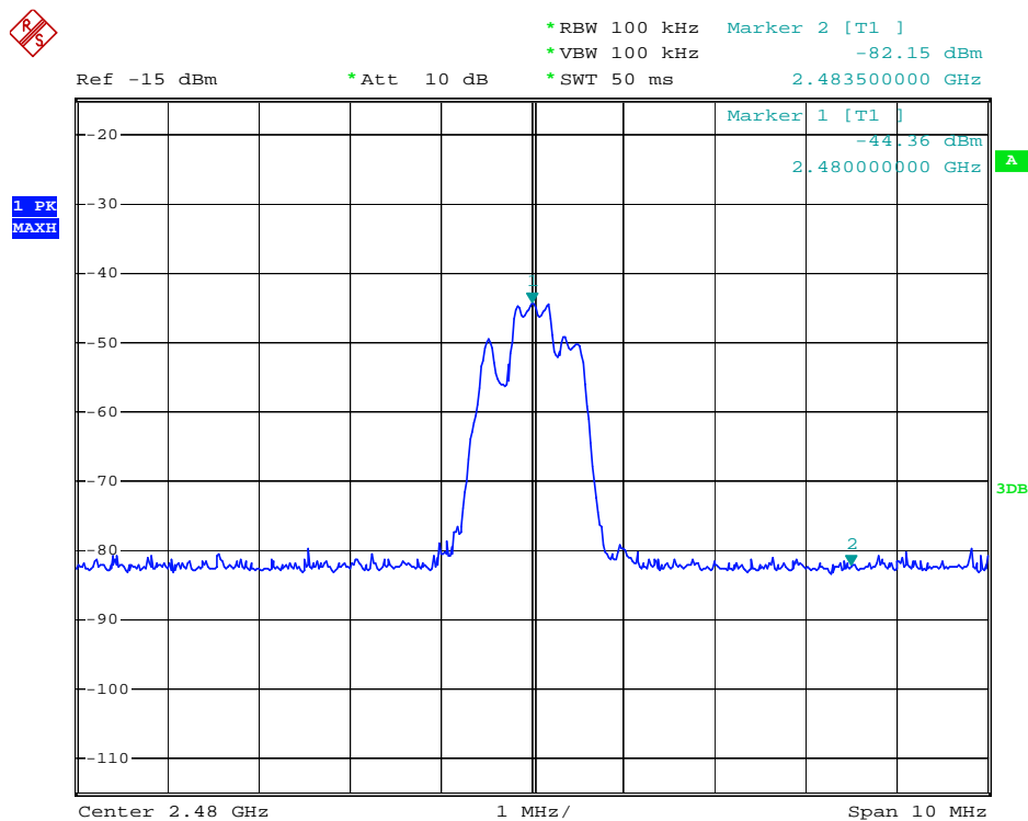
CH79_2480MHz
