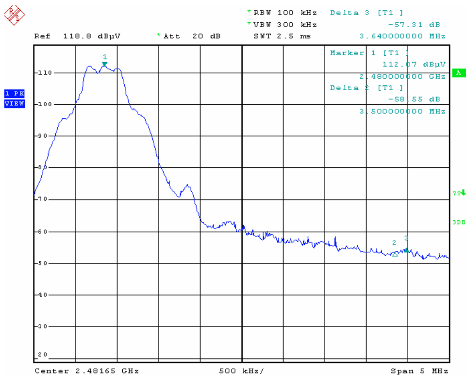
CH79_2480MHz
