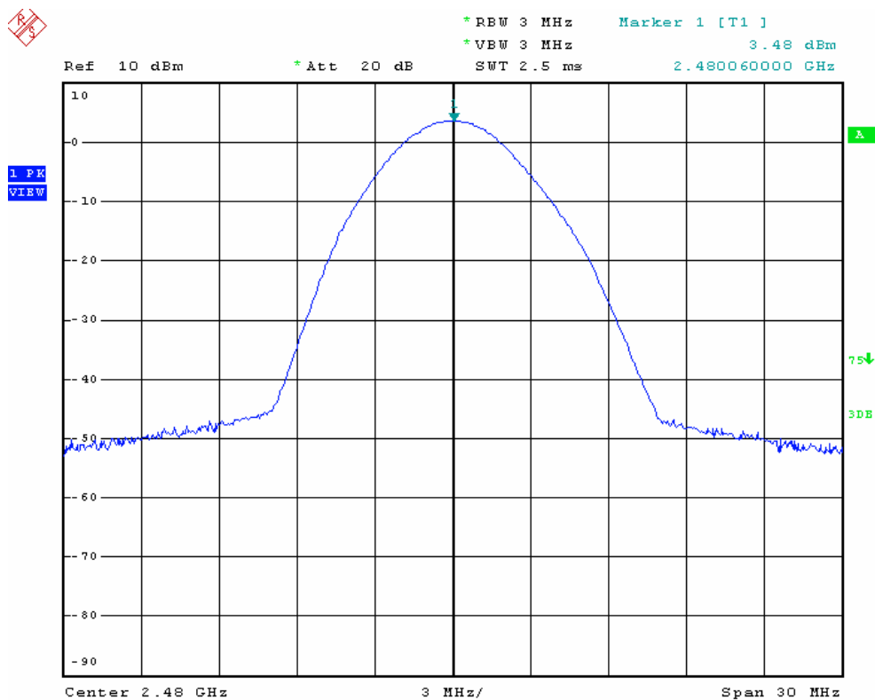
CH79_2480MHz
