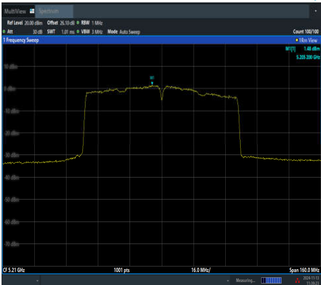
11AC80SISO-Ant3-5210-PASS
