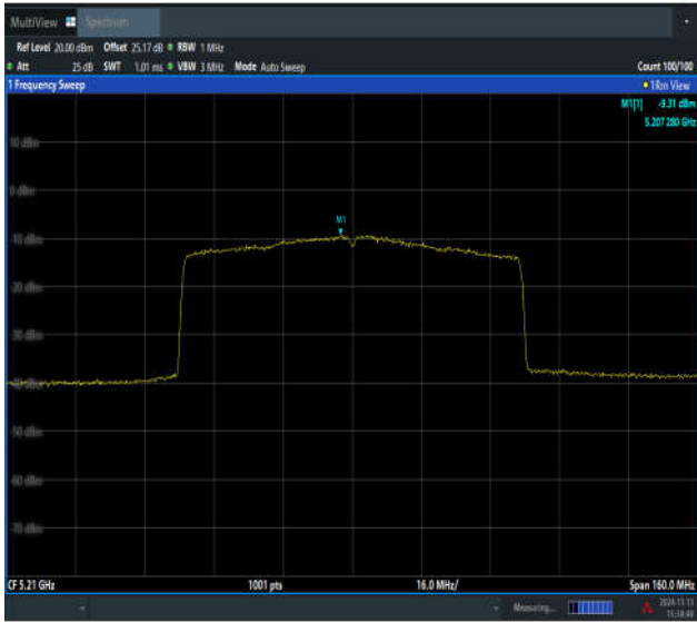
11AX80MIMO-Ant1-5210-PASS
