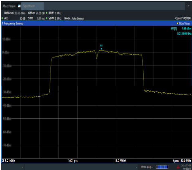
11AC80SISO-Ant2-5210-PASS
