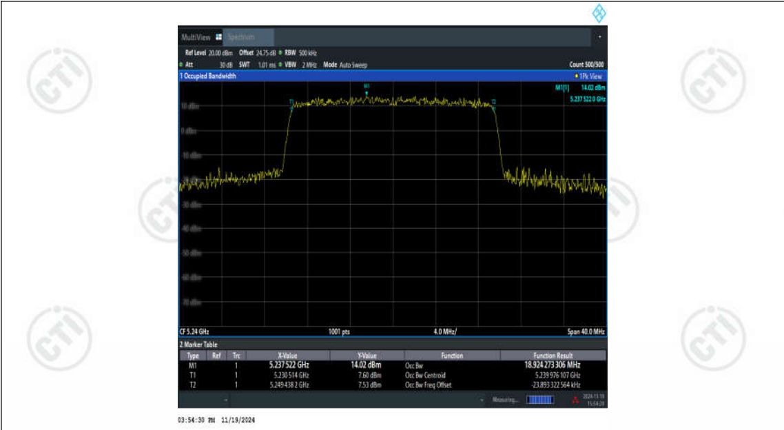
11BE20ISO-Ant3-5240
