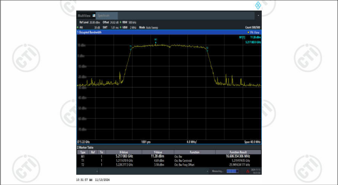
11A-Ant3-5220
