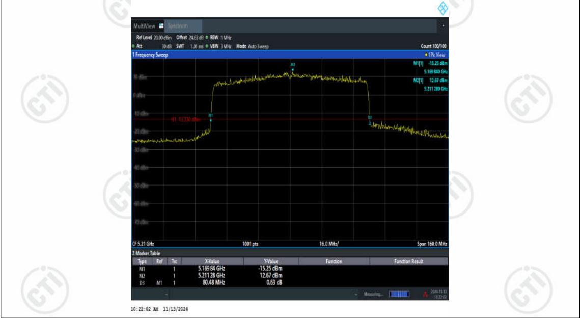
11AX80SISO-Ant2-5210
