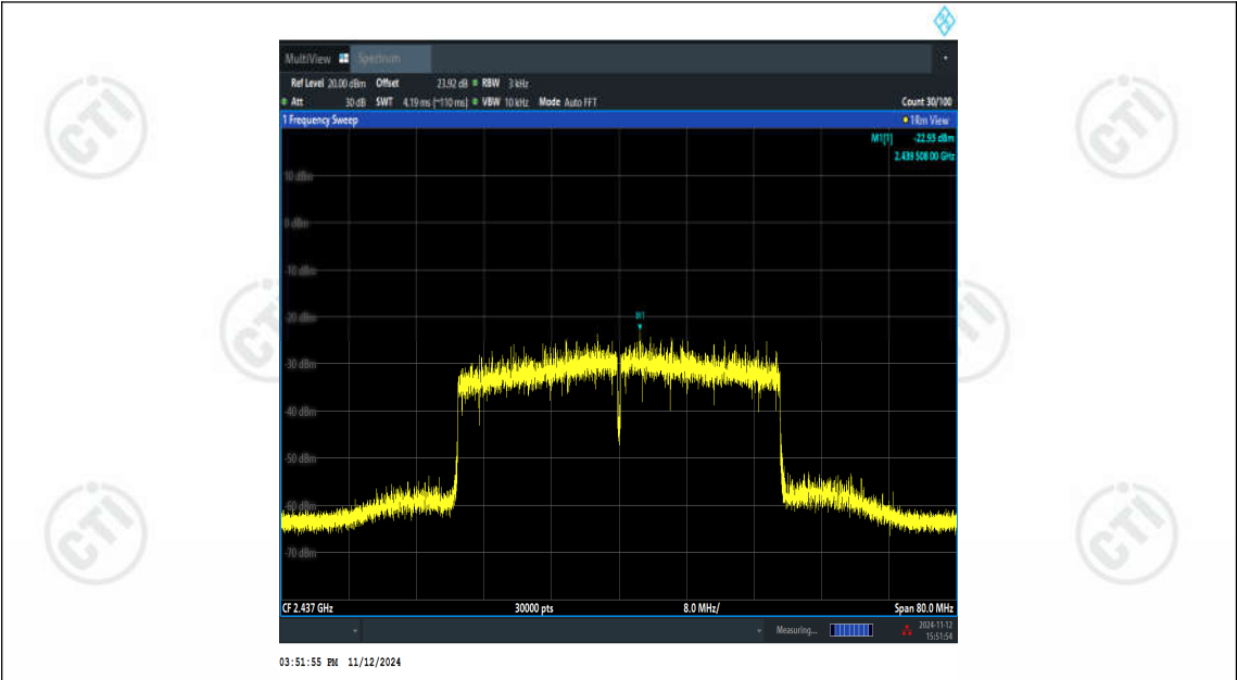
11AX40MIMO-Ant1-2437-PASS
