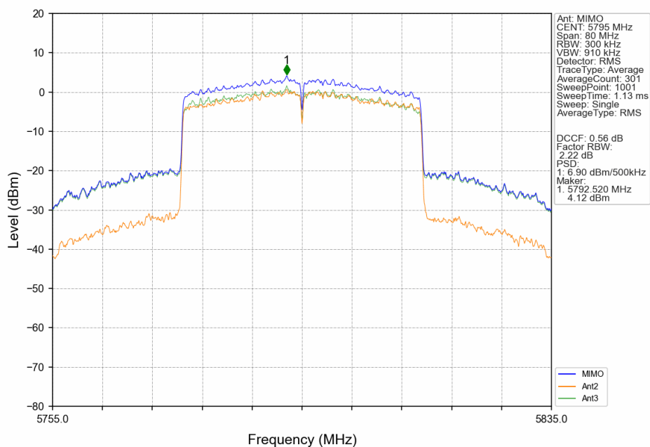
802.11be(EHT40)_HCH_5795MHz_SU_ / _MIMO_NTNV
