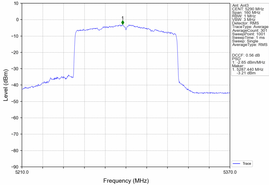
802.11be(EHT80)_MCH_5290MHz_SU_ / _MIMO_NTNV
