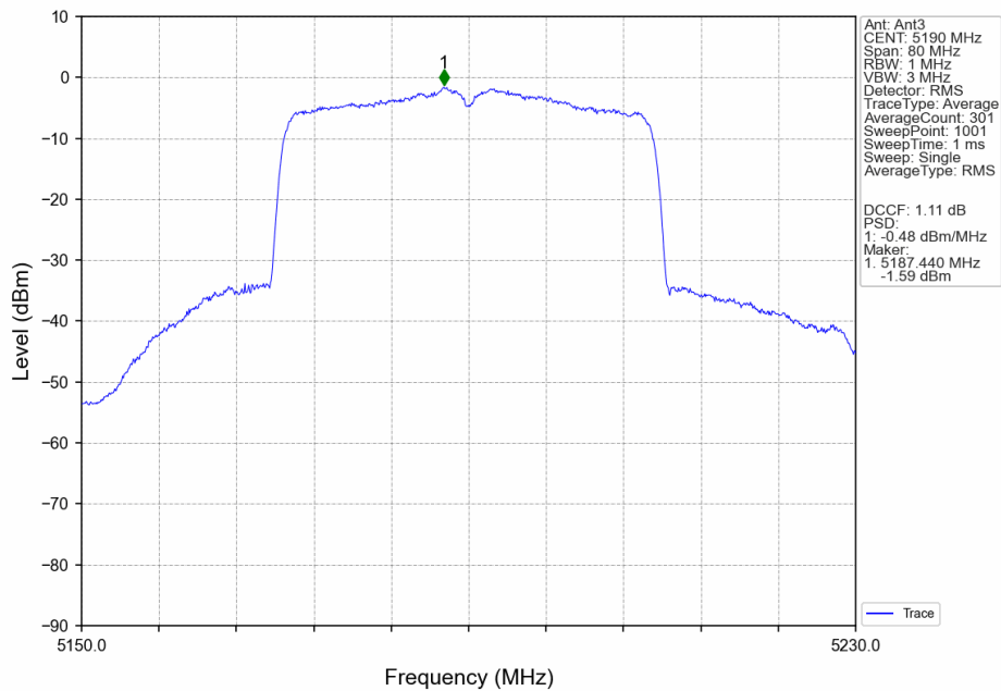
802.11be(EHT40)_LCH_5190MHz_SU_ / _Ant3_NTNV
