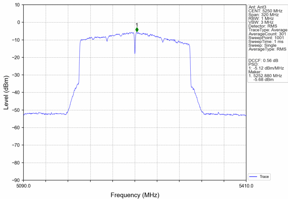
802.11be(EHT160)_MCH_5250MHz_SU_ / _Ant3_NTNV
