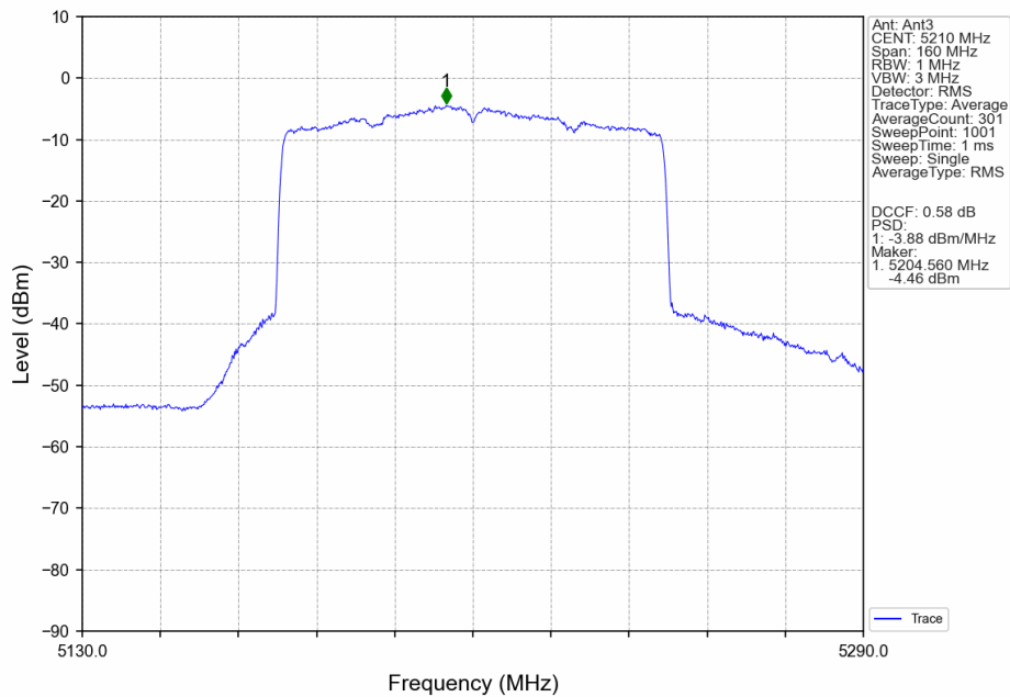
802.11be(EHT80)_MCH_5210MHz_SU_ / _Ant3_NTNV
