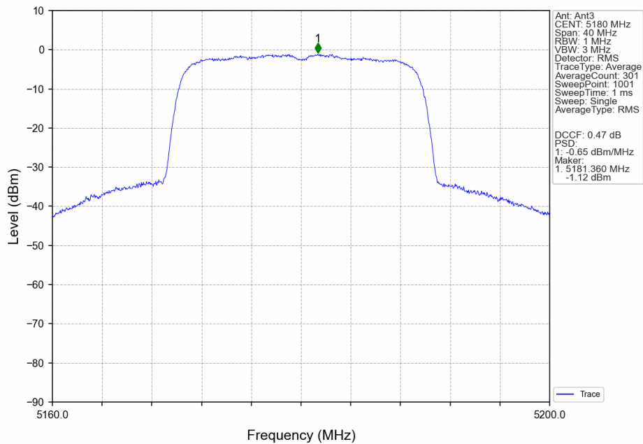
802.11be(EHT20)_LCH_5180MHz_SU_ / _Ant3_NTNV
