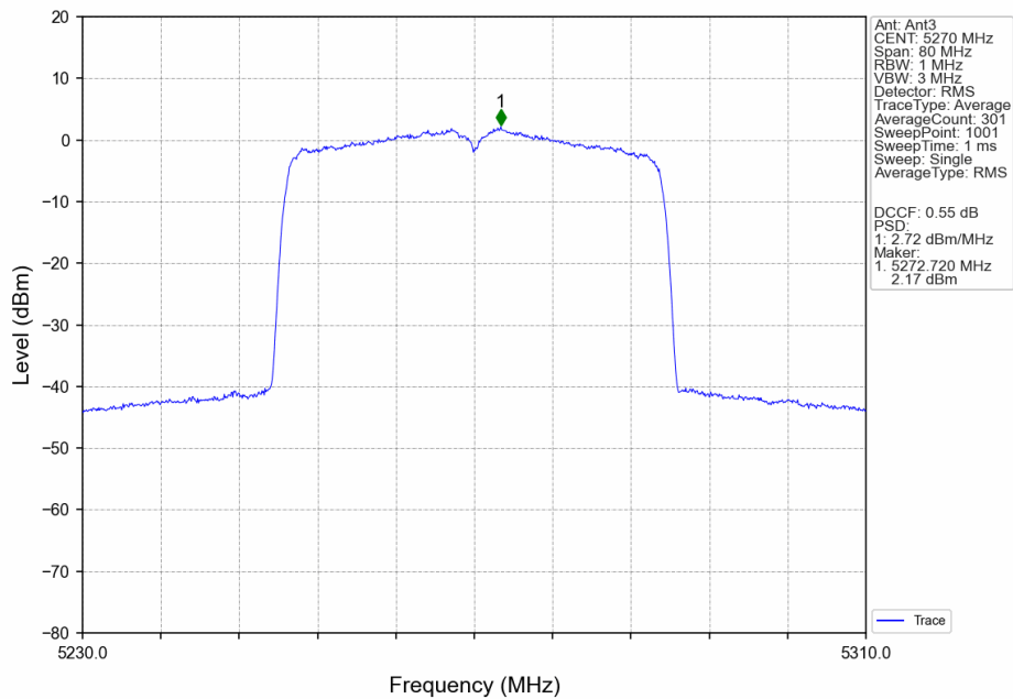
802.11be(EHT40)_LCH_5270MHz_SU_ / _Ant3_NTNV
