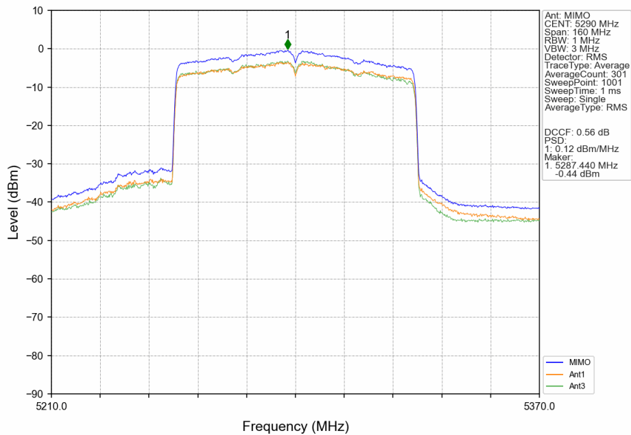
802.11be(EHT80)_MCH_5290MHz_SU_ / _MIMO_NTNV
