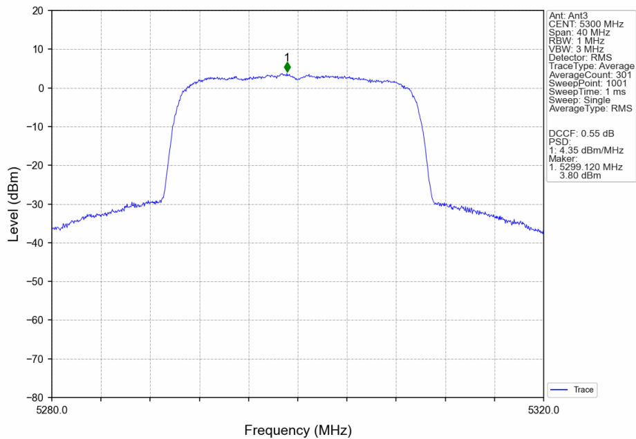
802.11be(EHT20)_MCH_5300MHz_SU_ / _Ant3_NTNV
