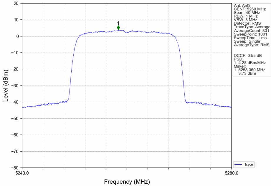
802.11be(EHT20)_LCH_5260MHz_SU_ / _MIMO_NTNV
