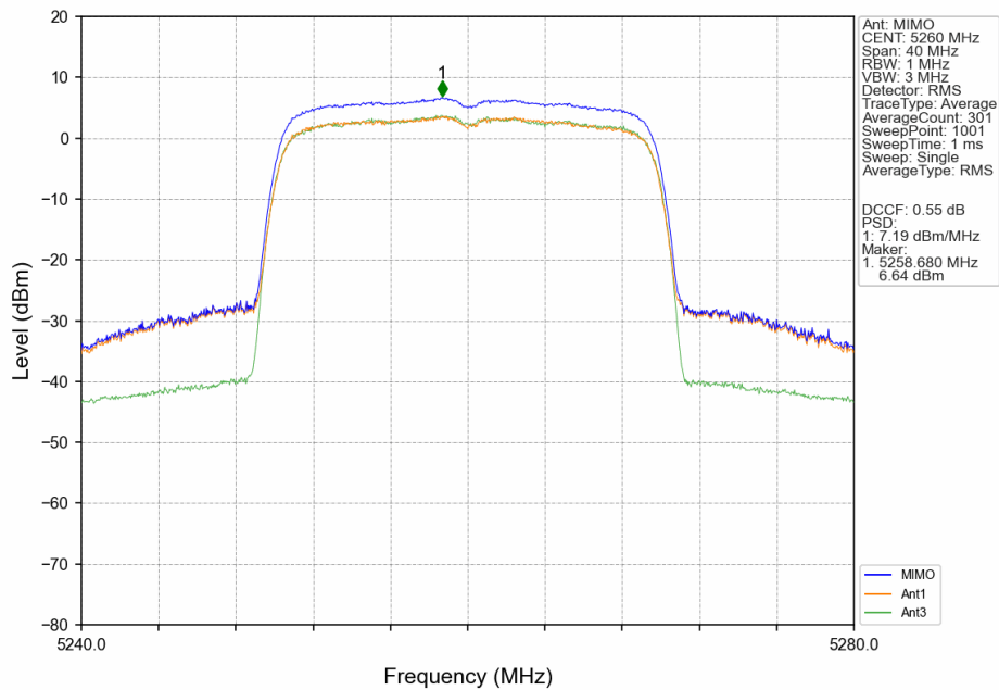
802.11be(EHT20)_LCH_5260MHz_SU_ / _MIMO_NTNV
