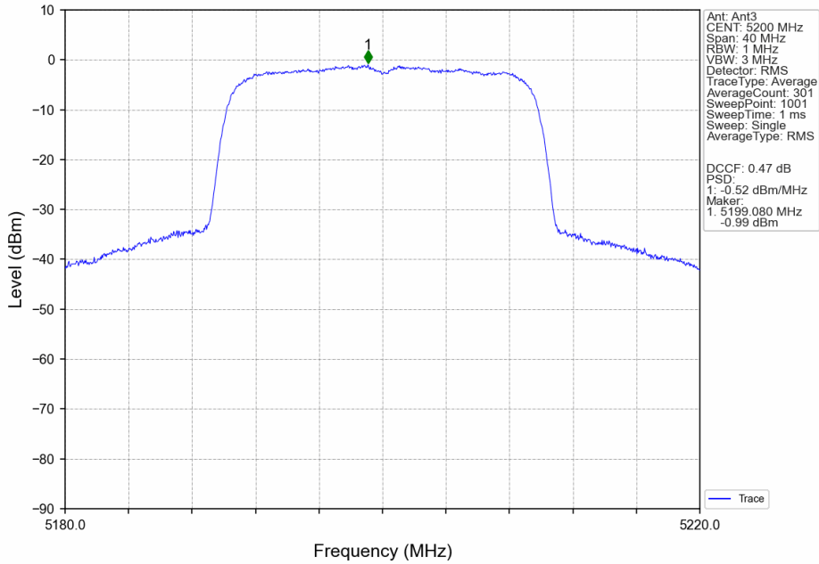
802.11be(EHT20)_MCH_5200MHz_SU_ / _MIMO_NTNV
