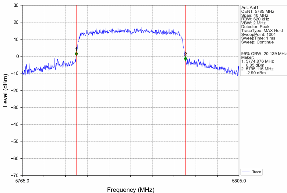
802.11be(EHT20)_MCH_5785MHz_SU_ / _Ant1_NTNV
