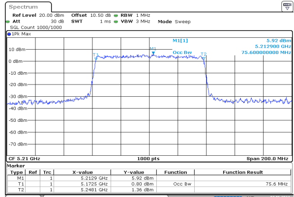
ac80_5210MHz_Chain 0
