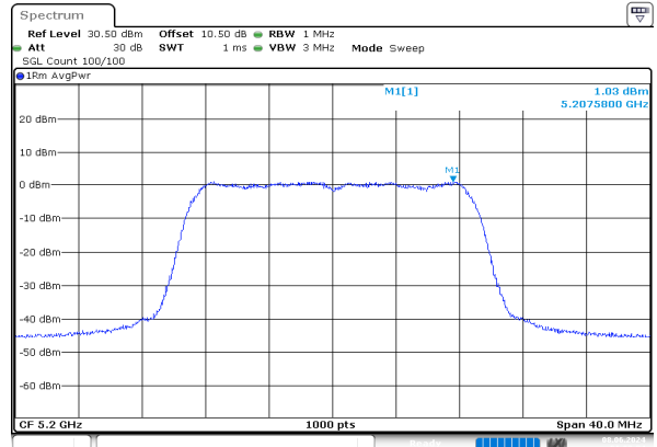
ac20_5200MHz_Chain 1
