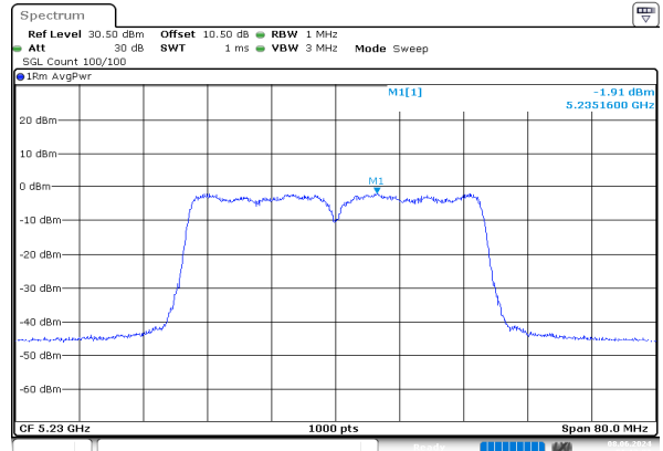
ac40_5230MHz_Chain 1
