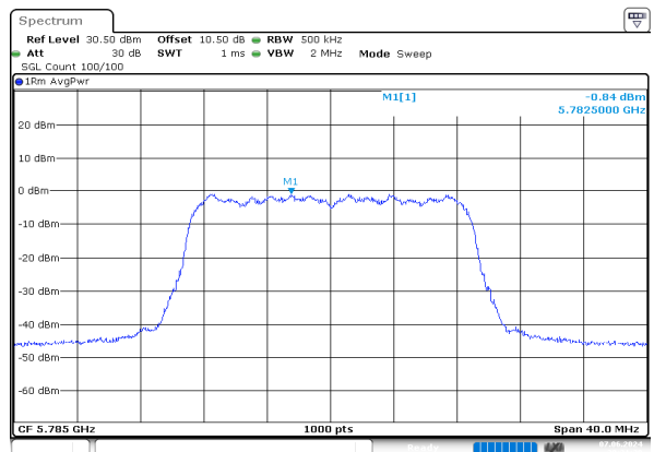
ac20_5785MHz_Chain 1
