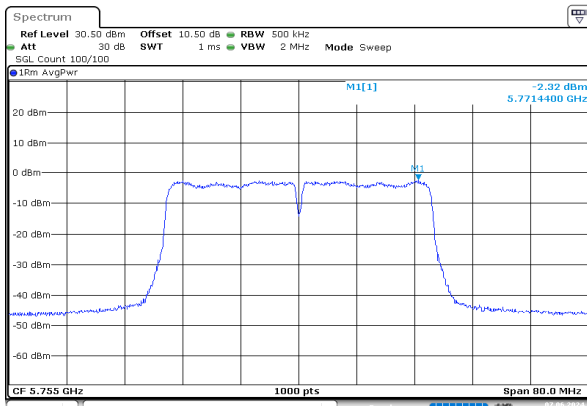
n40_5755MHz_Chain 0
