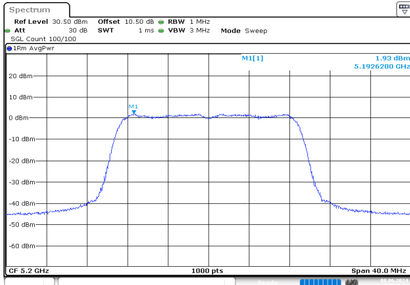
ac20_5200MHz_Chain 0
