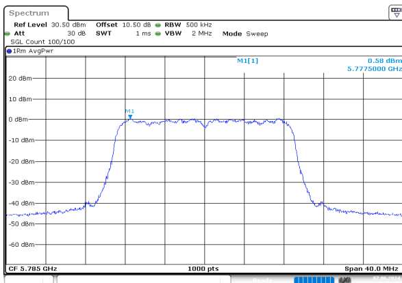
ac20_5785MHz_Chain 0
