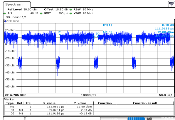
ac20_5785MHz_Chain 0
