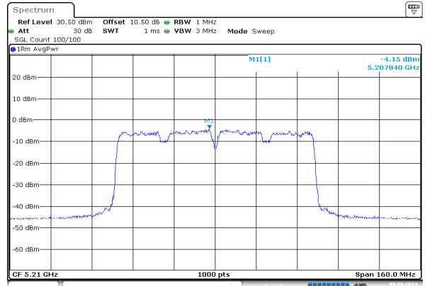
ac80_5210MHz_Chain 1
